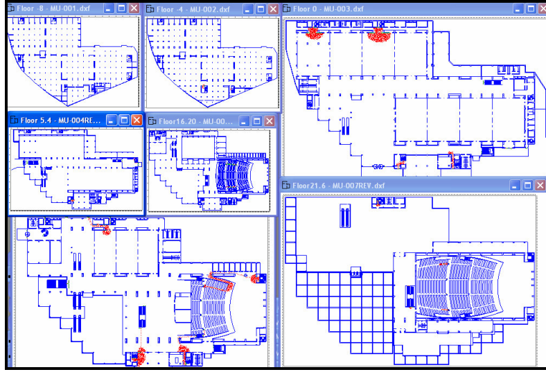
Şekil 4.23. 1. modellemede 5 dakikanın sonunda binada 4305 kişi bulunmaktadır. Binadan 5838 kişi ayrılmıştır.
