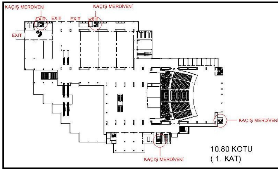
Şekil 4.12. +10.80 kotu planı ( Üst zemin kat planı)
