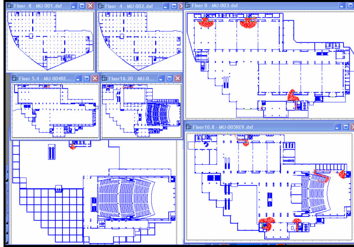
Şekil 4.44. 3. modellemeye 5. dakika sonunda binada 6359 kullanıcı bulunmaktadır.. Binadan 11242 kullanıcı ayrılmıştır
