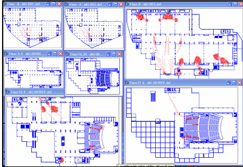
Şekil 4.21. 1. modellemede ilk 30 s sonunda binada 9670 kişi bulunmaktadır. Binadan 471 kişi ayrılmıştır.
