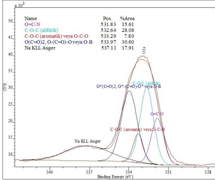
Şekil 1.11. 230 °C'ta sentezlenen BKKNT ürününe ait O1s pikinin bağlanma enerjisine karşılık gelen kaymalar
