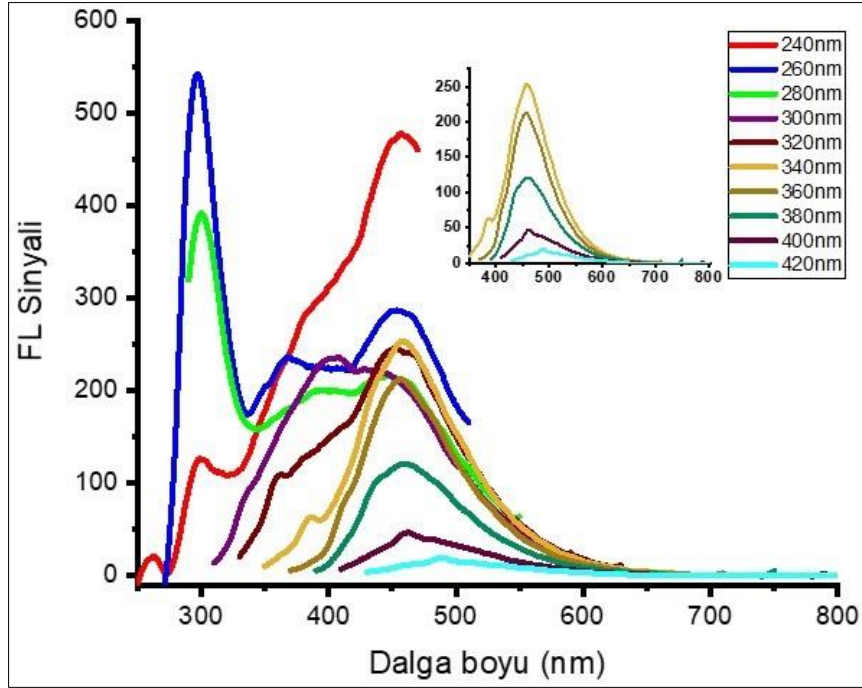
Şekil 4.9. 230 °C'ta sentezlenen BKKNT ürününün uyarma dalga boyuna bağlı olarak FL emisyonunda meydana gelen kaymalar (iç grafik: 340-420 nm arası uyarıma bağlı olarak FL emisyonunda meydana gelen değişim)
