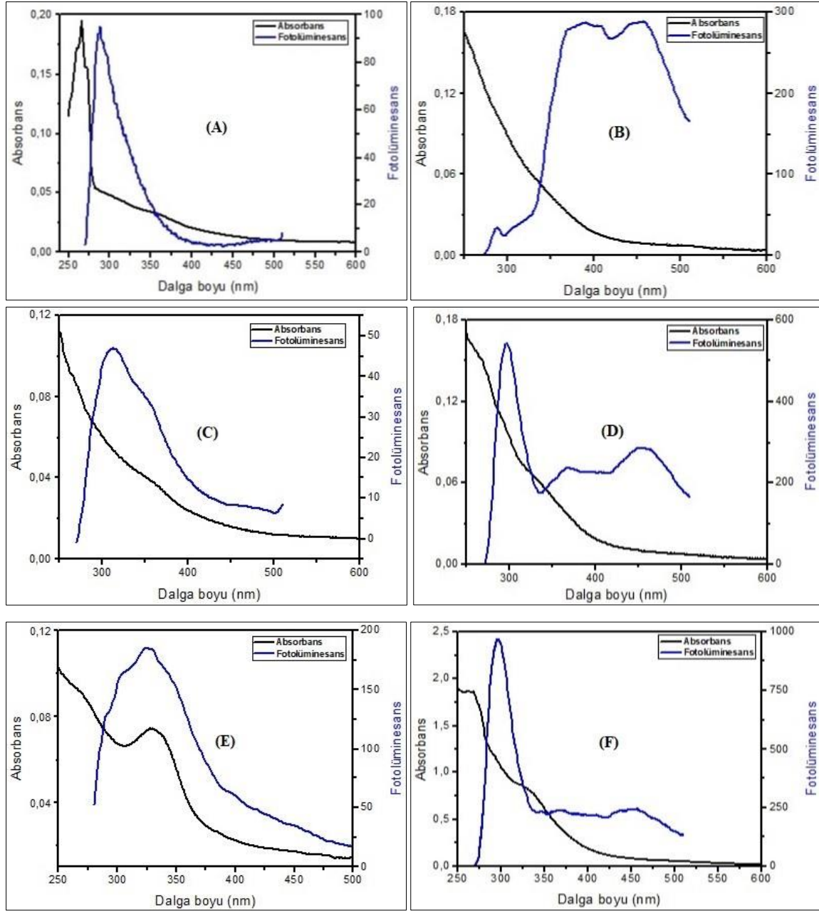
Şekil 4.7. (A) 170 °C (B) 190 °C (C) 210 °C (D) 230 °C (E) 250 °C ve (F) 270 °C’ta sentezlenen BKKNT ürünlerinin UV-GB absorbans ve maksimum FL şiddetinin alındığı emisyon spektrumlarının üst üste çakıştırılmış hali
