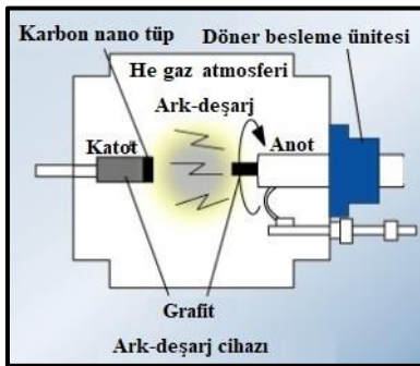
Şekil 2.4. Ark deşarj cihazının şematik gösterimi
