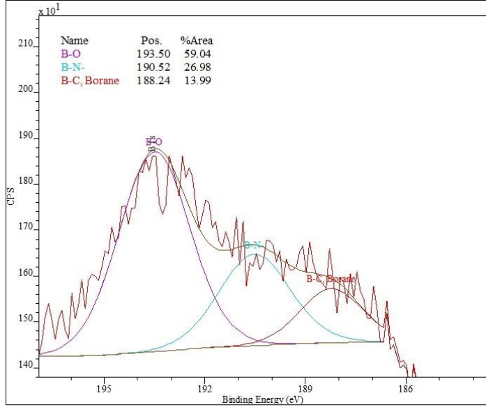
Şekil 1.9. 230 °C'ta sentezlenen BKKNT ürününe ait B1s pikinin bağlanma enerjisine karşılık gelen kaymalar
