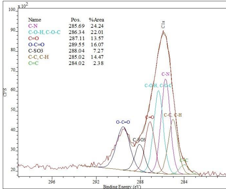
Şekil 1.2. 190 °C'ta sentezlenen BKKNT ürününe ait C1s pikinin bağlanma enerjisine karşılık gelen kaymalar
