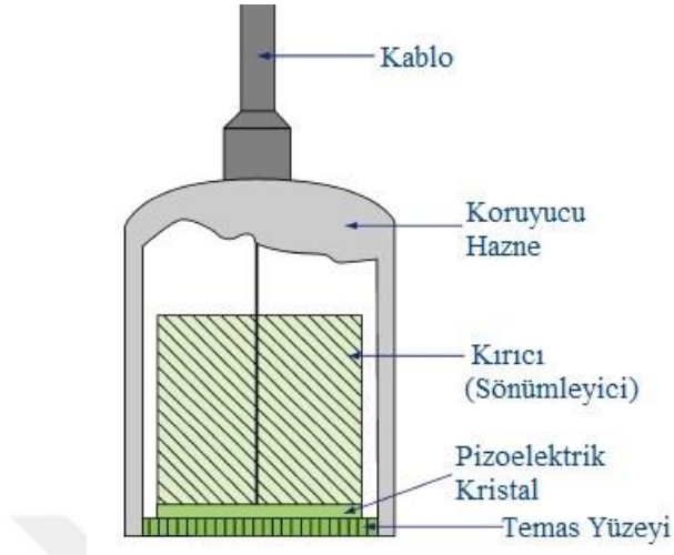
Şekil 14 Ultrason Dönüştürücüsünün (Probun) Yapısı
