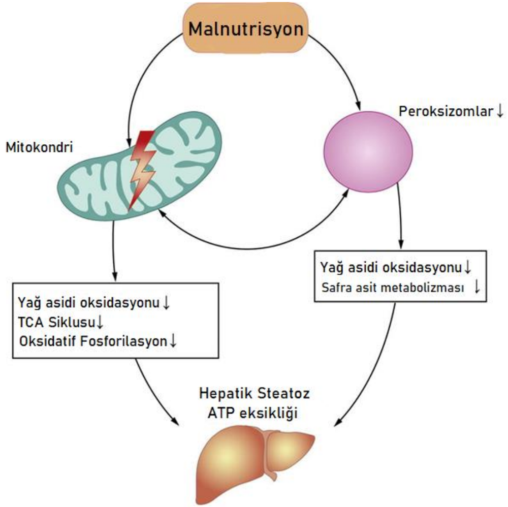
Şekil 12 Düşük protein içerikli diyetin neden olduğu hepatik peroksizom kaybı ve mitokondriyal disfonksiyon modeli
