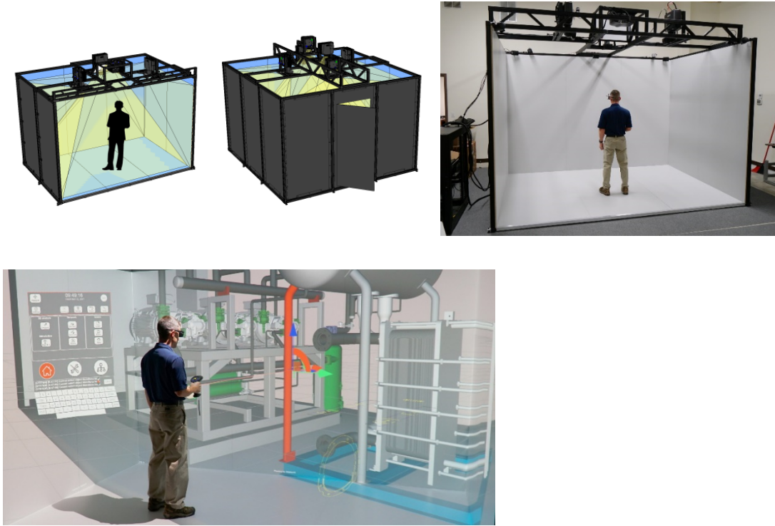
Resim 2.3. VisCube™ M4 CAVE sistemi (Visbox, t.y.)
