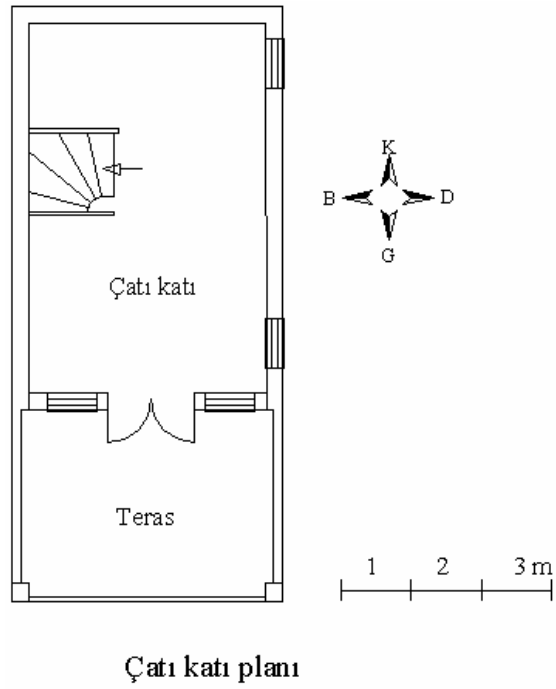
Şekil 2.26. On altı numaralı ev planı [Gümüş, 2006]
