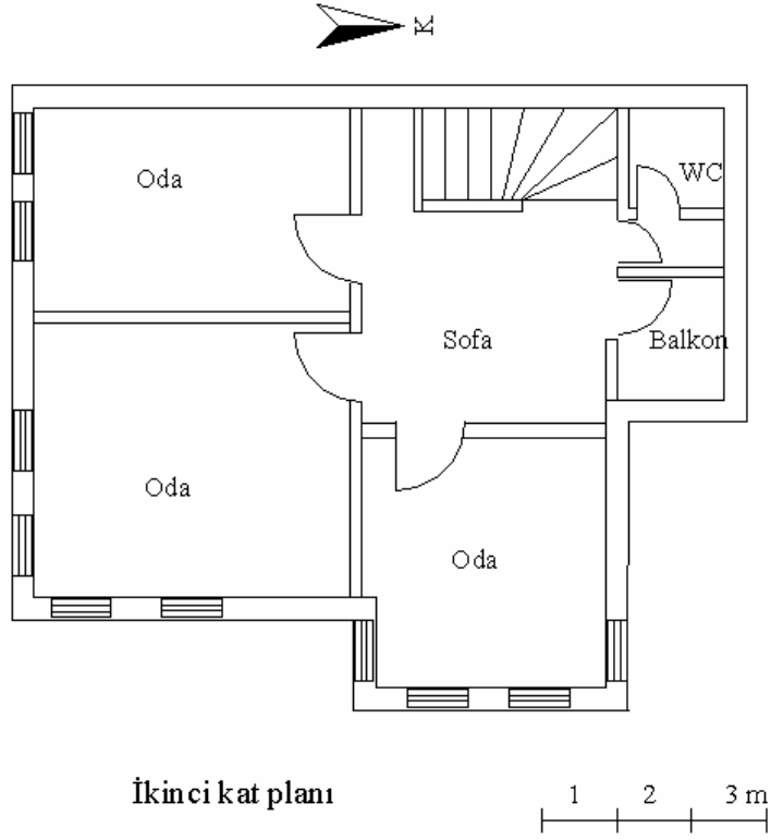
Şekil 2.4. İki numaralı evin planı [Gümüş, 2006]
