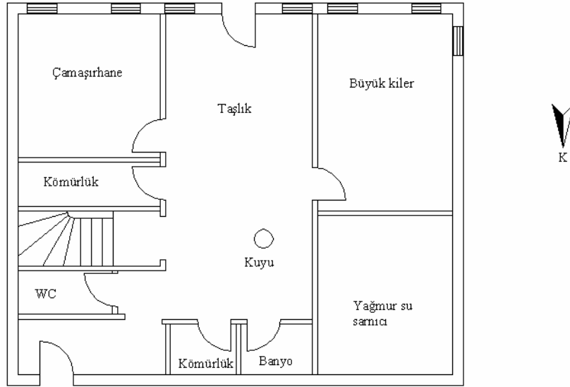
Zemin kat planı
