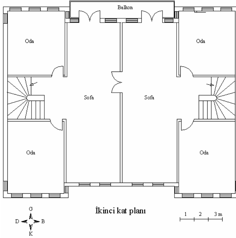
Şekil 2.19. On bir numaralı ev planı [Gümüő, 2006]
