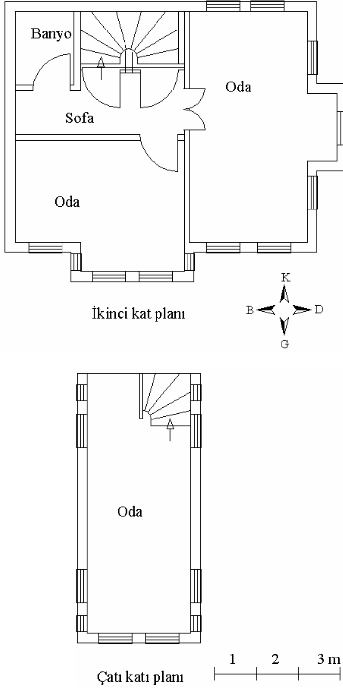
Şekil 2.28. On yedi numaralı ev planı [Gümüş, 2006]
