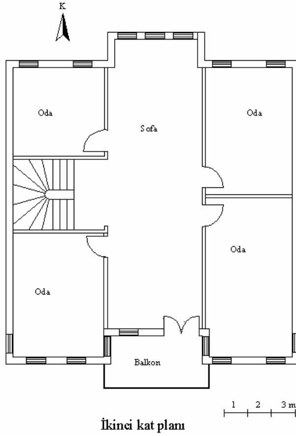
Şekil 2.6. Üç numaralı evin planı [Gümüş, 2006]
