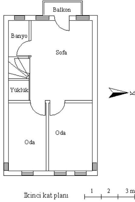
Şekil 2.10. Beş numaralı ev planı [Gümüş, 2006]
