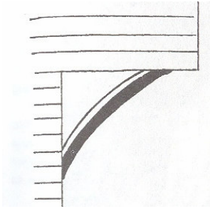
Şekil 2.2 Dört köşe kesitli, eğri ağaç (eli böğründe) [Satkın,1996]
