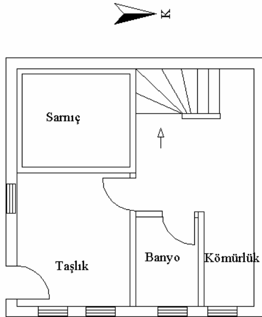
Zemin kat planı
