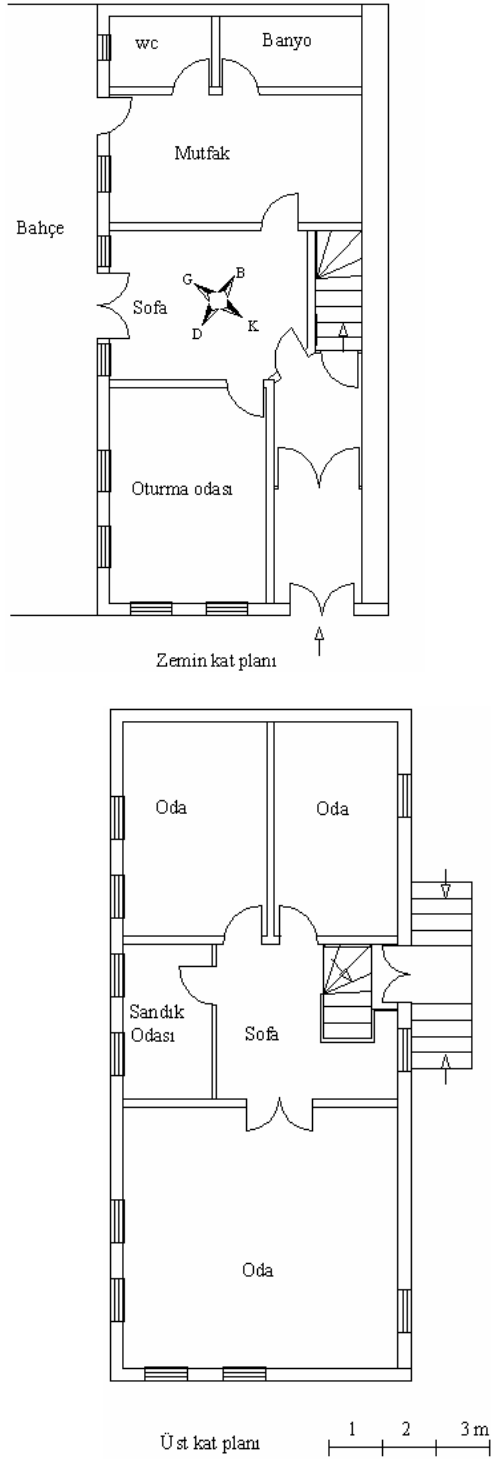
Şekil 2.15. Dokuz numaralı ev planı [Gümüş, 2006]
