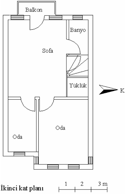
Şekil 2.12. Altı numaralı ev planı [Gümüş, 2006]
