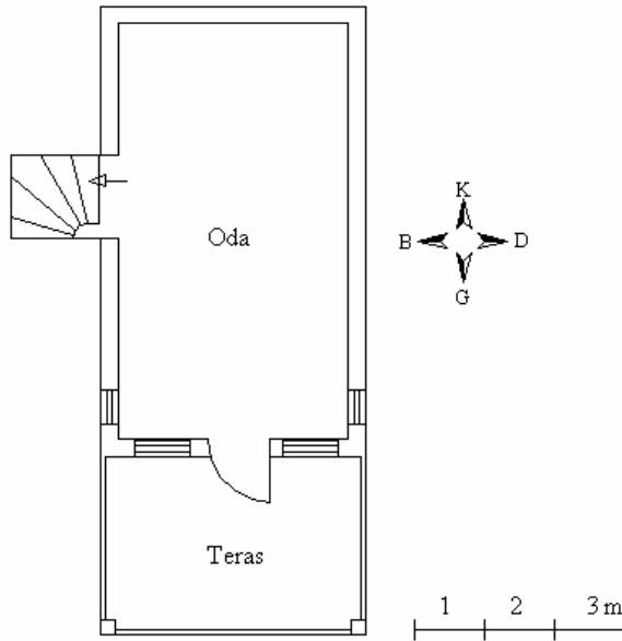
Çatı katı planı
