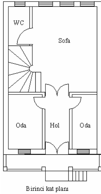
Şekil 2.9. Beş numaralı ev planı [Gümüş, 2006]
