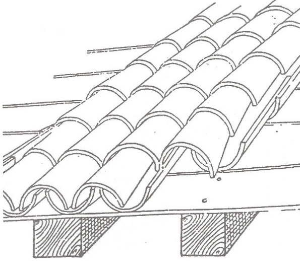
Şekil 2.9 Osmanlı kiremidi ve diziliş şekli [Satkın,1996]
