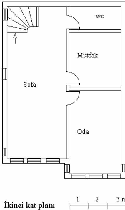
Şekil 2.16. On numaralı ev planı [Gümüş, 2006]
