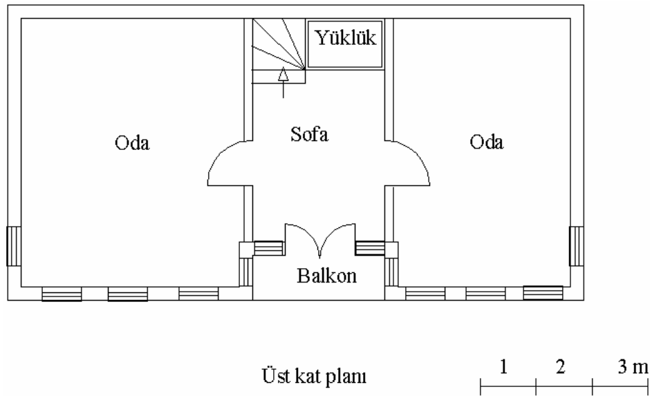
Şekil 2.24. On dört numaralı ev planı [Gümüş, 2006]
