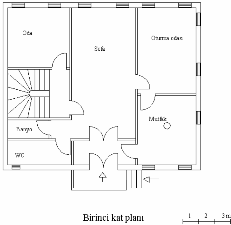
Şekil 2.1. Bir numaralı evin planı [Gümüş, 2006]
