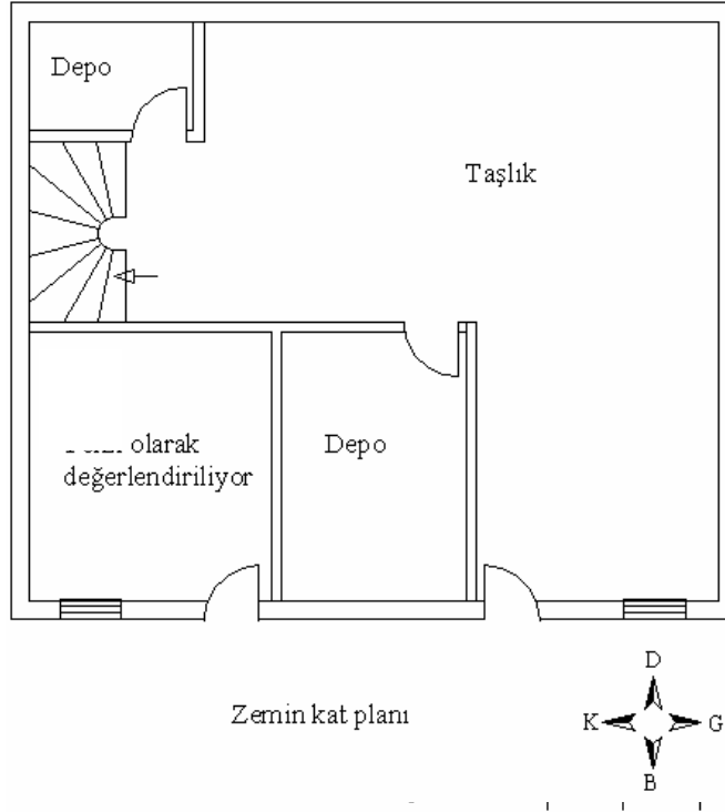
Şekil 2.29. On sekiz numaralı ev planı [Gümüş, 2006]
