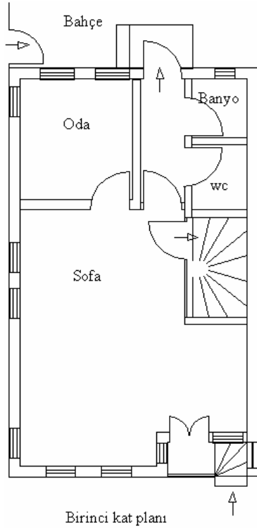
Şekil 2.20. On iki numaralı ev planı [Gümüş, 2006]
