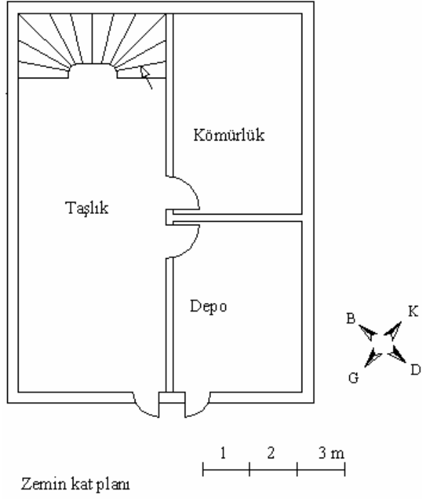
Şekil 2.17. On numaralı ev planı [Gümüş, 2006]
