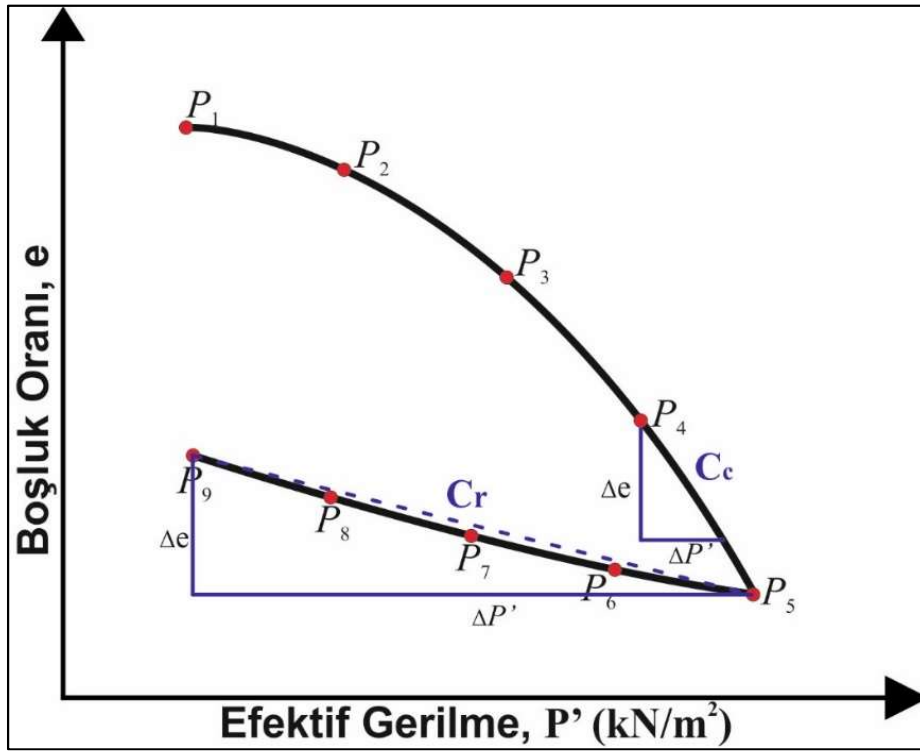
Şekil 3.5. Tekrar sıkışma indisinin belirlenmesi
