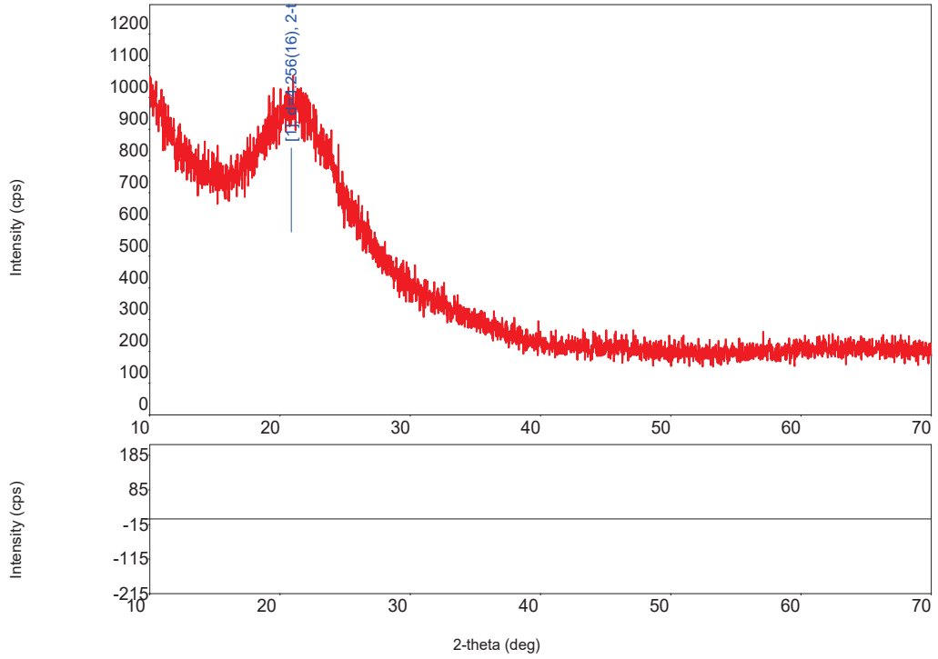
Şekil 6.14 . %6 \text{Cr}(\text{NO}_3)_3 /TEOS içeren İnce Filmin XRD Spektrumu
