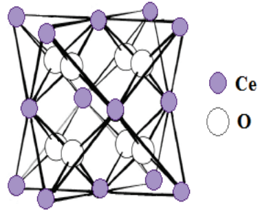
Şekil 5.2. Seryum Oksidin Kristal Yapısı[40]
