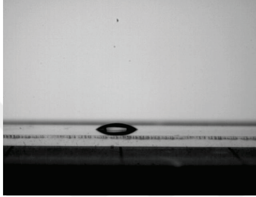
Resim 6.1. Kaplama yapılmamış cam yüzeyin temas açısı
