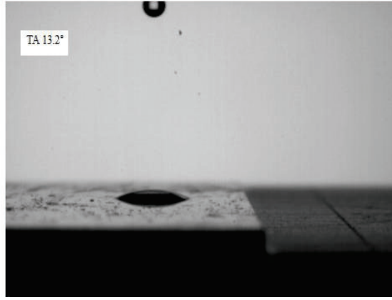
Resim 6.3. %4 \text{Cr}(\text{NO}_3)_6 /TEOS ile kaplanan cam yüzeyin temas açısı
