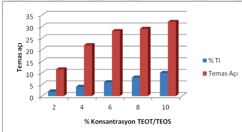
Şekil 6.4. Temas açısının TEOT/TEOS miktarı ile değişimi
