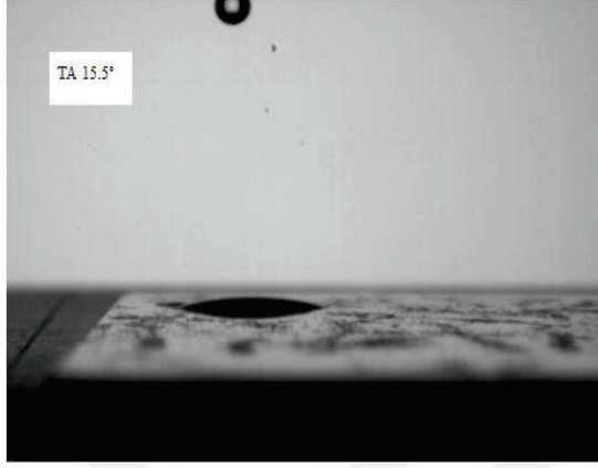
Resim 6.4. %6 \text{Cr}(\text{NO}_3)_3 /TEOS ile kaplanan cam yüzeyin temas açısı
