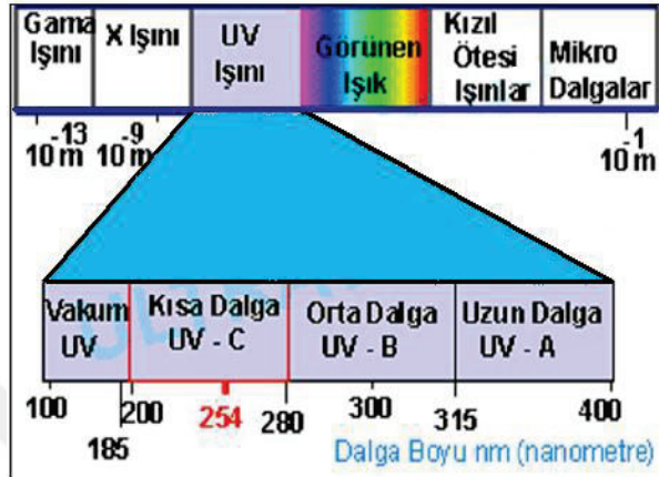
Çizelge 2.1. UV ışınlarının dalga boyu aralıkları
