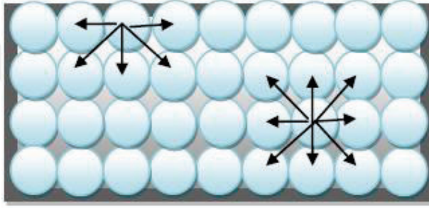
Şekil 2.12.Sıvı molekülleri ve aralarındaki etkileşim kuvvetleri
