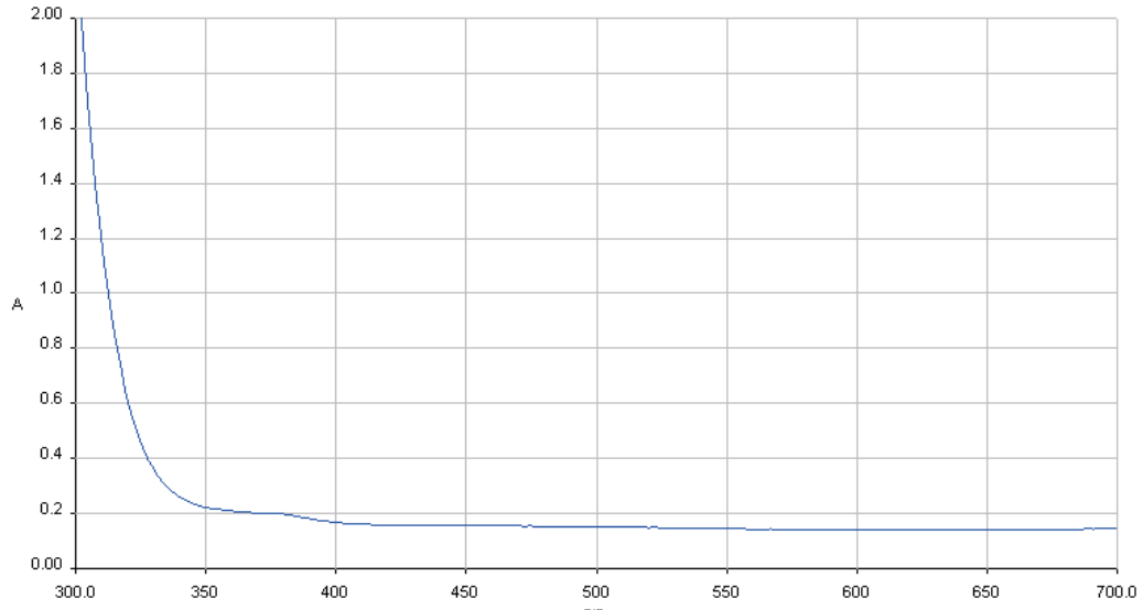
Şekil 6.8. %8 Cr(NO 3 ) 3 /TEOS 370 nm absorpsiyonu
