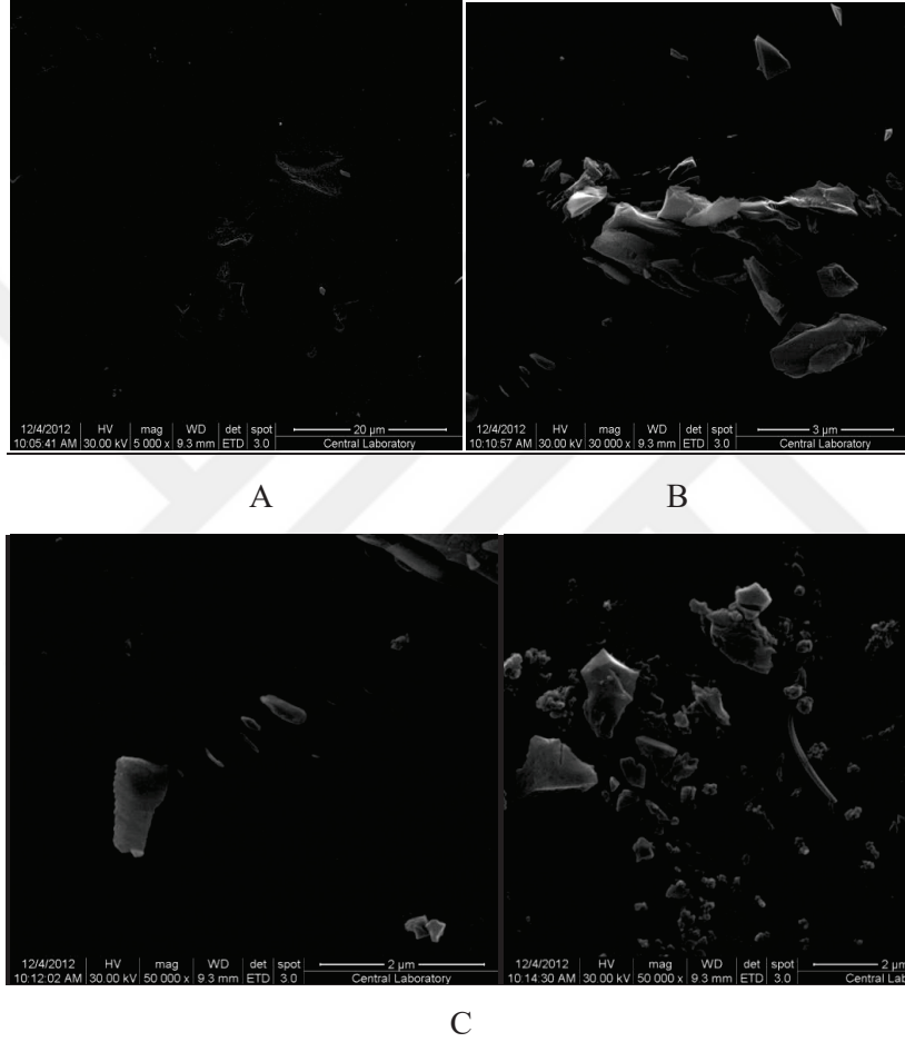
Resim 6.13. % 6 TEOT / TEOS kaplı örneklerin SEM görüntüleri
