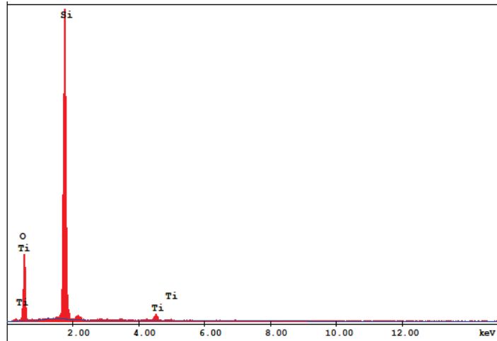
Şekil 6.7. %6 TEOT/ TEOS kaplı örneklerin EDS spektrasi
