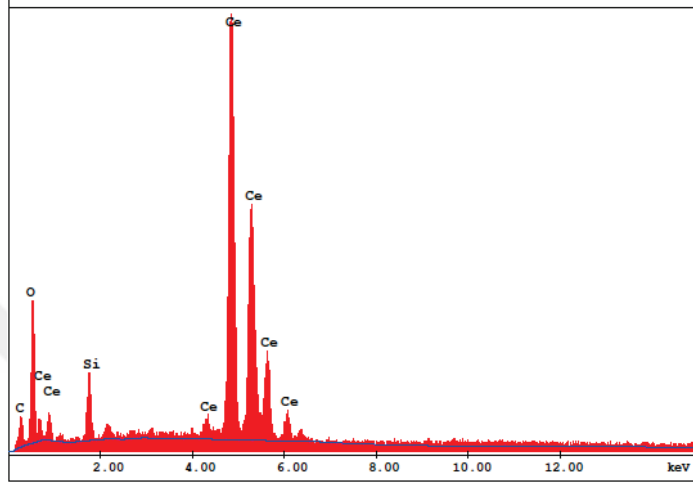
Şekil 6.6. %6 CeO 2 / TEOS kaplı örneklerin EDS spektrasi
