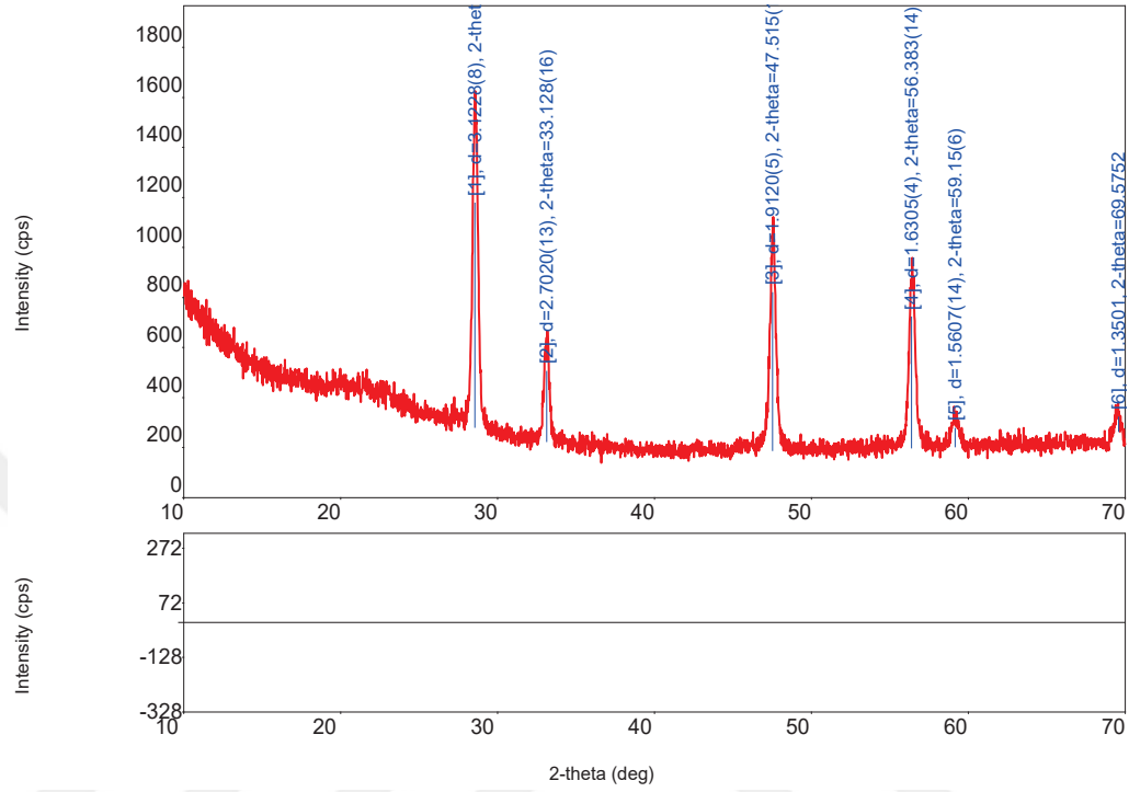
Şekil 6.15 . %6 CeO 2 /TEOS içeren İnce Filmin XRD Spektrumu
