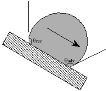
Şekil 2.11. İlerleyen ve gerileyen temas açılarının hareketi[49]
