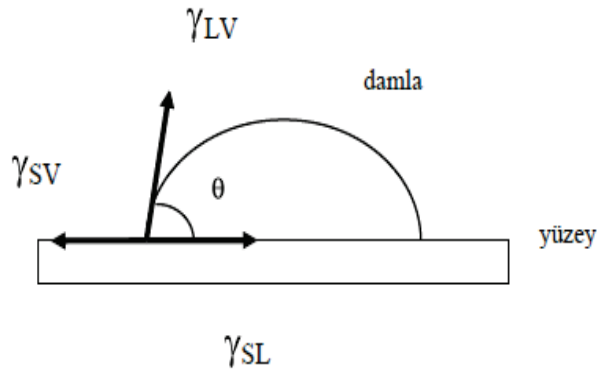
Şekil 2.10. Denge temas açısında yüzey enerjisi bileşenleri[46]
