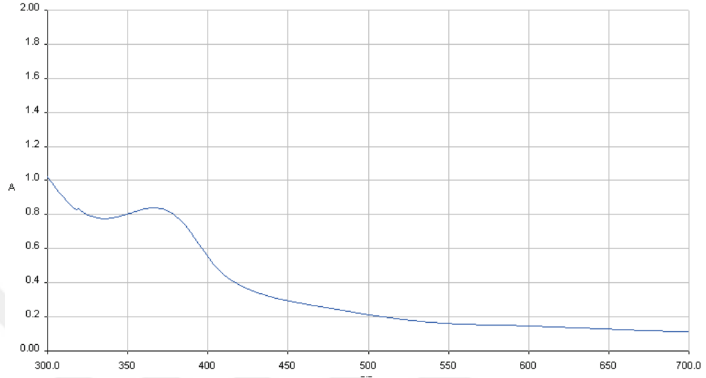
Şekil 6.11. %8 \text{Cr}(\text{NO}_3)_3 370 nm absorpsiyonu
