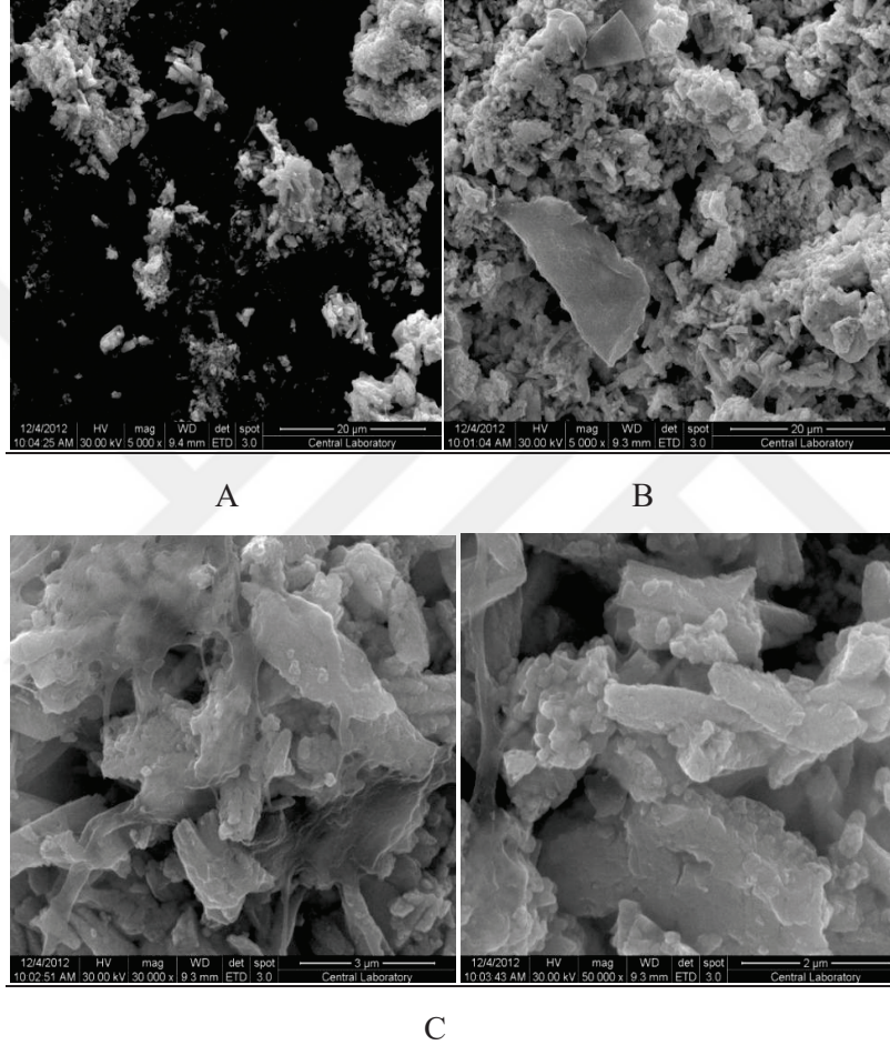
Resim 6.12. % 6 CeO 2 / TEOS kaplı örneklerin SEM görüntüleri
