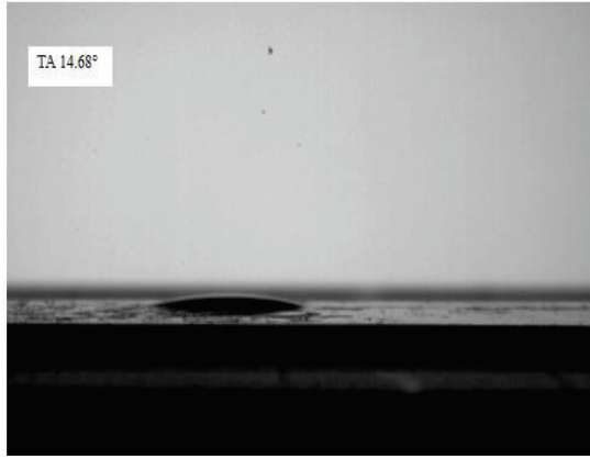
Resim 6.5. %8 \text{Cr}(\text{NO}_3)_3 /TEOS ile kaplanan cam yüzeyin temas açısı
