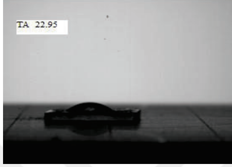
Resim1.1. %2 CeO 2 /TEOS ile kaplanan cam yüzeyin temas açısı
