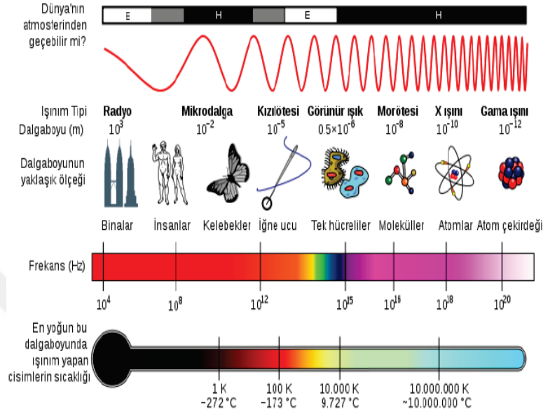
Şekil 2.8. Elektromanyetik spektrumdaki ışınlar, dalga boyları, frekansları ve en yoğun dalga boyunda ışıyan cisimlerin sıcaklığı
