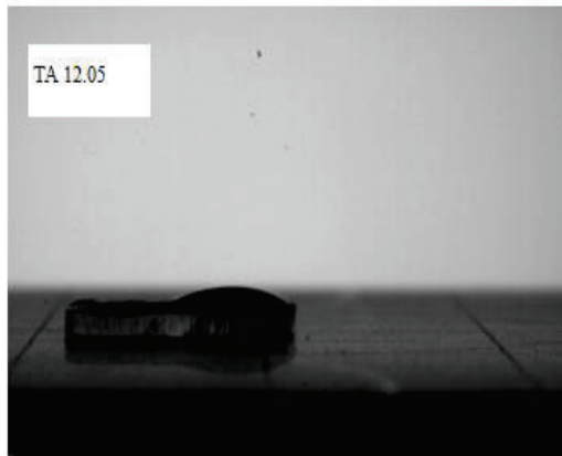
Resim 6.8. % 6\text{CeO}_2/\text{TEOS} ile kaplanan cam yüzeyin temas açısı
