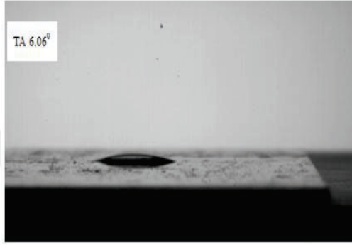
Resim 6.2. %2 \text{Cr}(\text{NO}_3)_6 /TEOS ile kaplanan cam yüzeyin temas açısı
