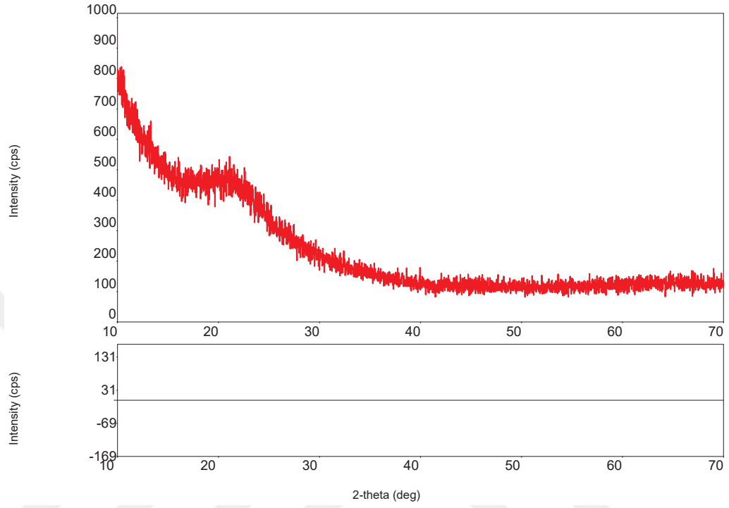
Şekil 6.13 .%6 TEOT/TEOS içeren İnce Filmin XRD Spektrumu
