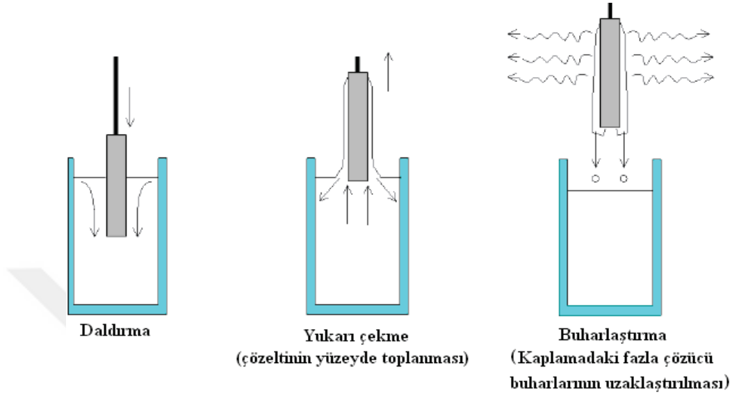
Şekil 2.5. Daldırma ile kaplama tekniği
