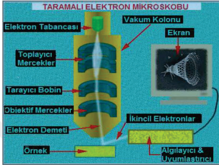
Şekil 2.7. Taramalı elektron mikroskobu( SEM)'nin şematik gösterimi [43]
