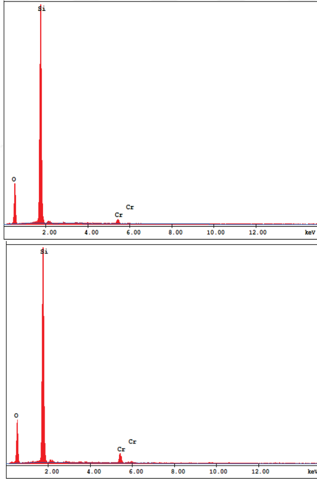
Şekil 6.5. %6 Cr (NO 3 ) 6 / TEOS kaplı örneklerin EDS spektralleri
