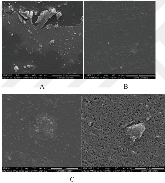
Resim 6.10. %6 \text{Cr}(\text{NO}_3)_6 / TEOS kaplı örneklerin SEM görüntüleri
