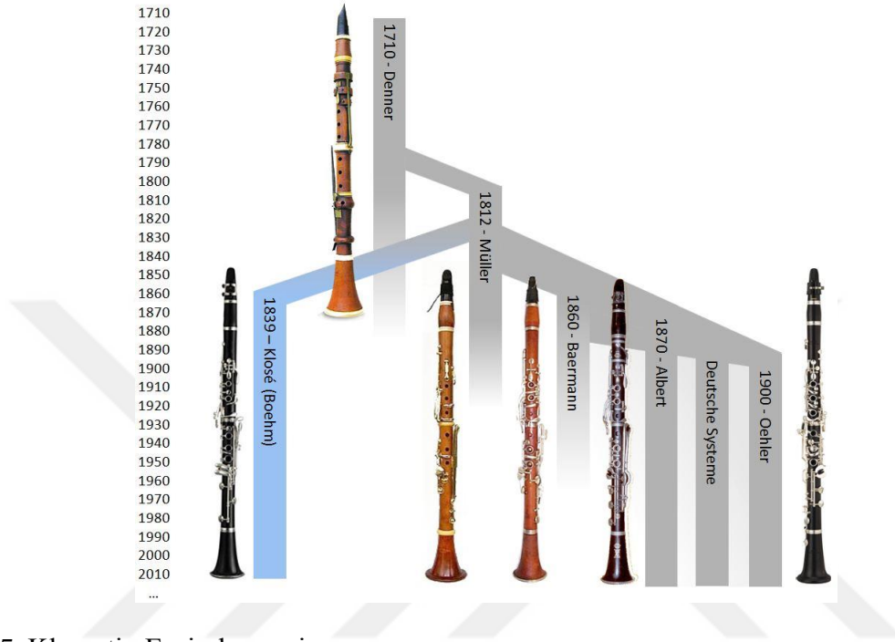
Şekil 5. Klarnetin Evrimleşmesi
