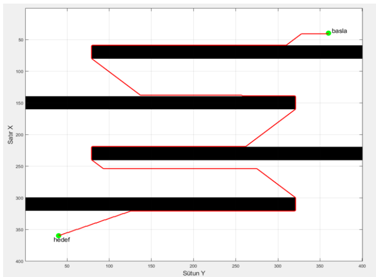
Şekil 5.23. Senaryo-8 haritası için A* algoritmasının oluşturduğu rota
