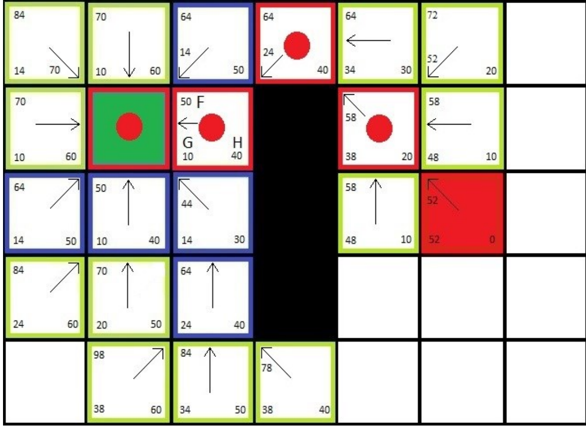
Şekil 4.12. Tarama sonunda yolun bulunması
