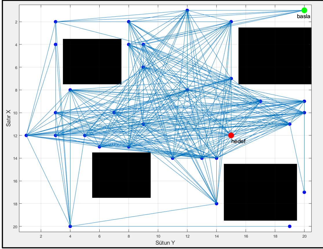
Şekil 4.21. PRM algoritmasının oluşturduğu yol haritası örneği
