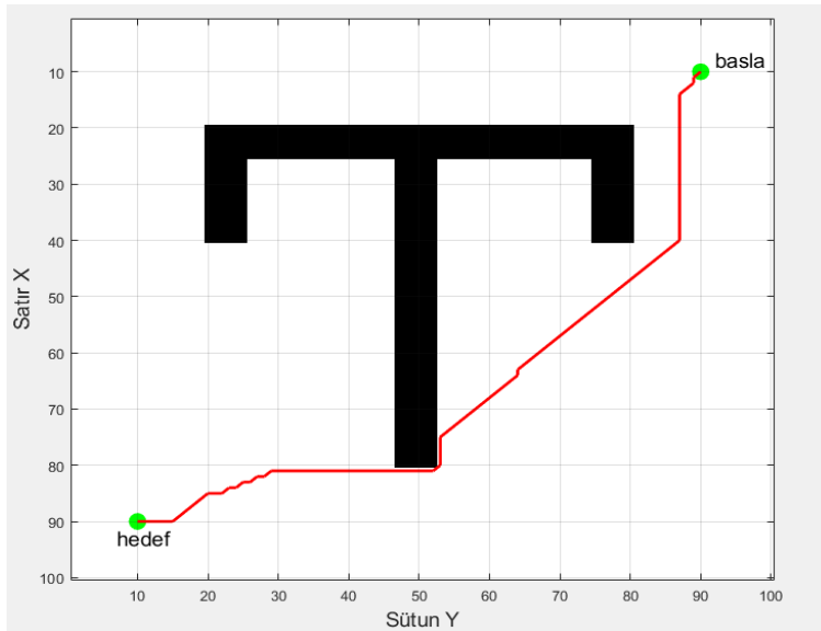
Şekil 5.2. Senaryo-1 haritası için A* algoritmasının oluşturduğu rota
