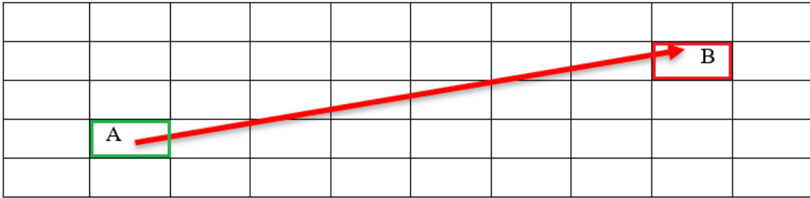
Şekil 4.1. 2 nokta arasındaki Öklid uzunluğu
