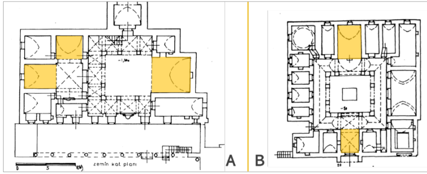
Şekil 2.70. Diyarbakır Mesudiye (A) ve Zinciriye (B) medreseleri planı (Altun, 1973)
