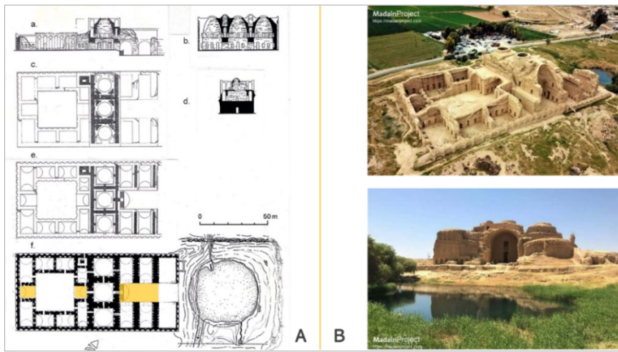
Resim 2.6. Firuzabad Ateşgedesi (I. Ardeşir'in Sarayı) A: (Huff, 2008) a. Eksenel uzunlamasına kesit; b. Üç kubbeden enine kesit; c. Yaşam alanı ikinci kat seviyesi; d. Boyuna kesit; e. Birinci kat planı; f. Zemin kat planı B: (Palace of Ardashir, 2022)
