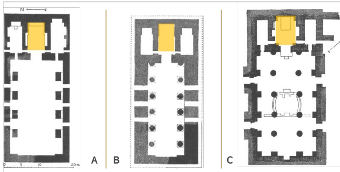
Şekil 2.30. Ktesifon (A,B) ve Hira'da (C) bulunan Sasani Dönemi Kiliseleri, (Hoddinott, 1963: 36–37)
