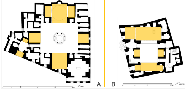
Şekil 2.120. Emir Sargıtmış (A) ve Emir Mitkal Anuki Medresesi (B), (Archnet, 2003)
