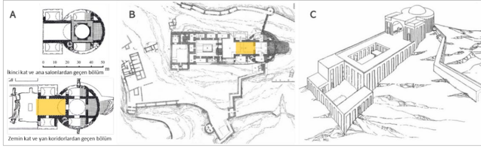
Şekil 2.21. Kale-i Duhtar, Eyvan ve kubbeli bölüm planı (A), (Huff, 2008) Plan ve perspektif (B,C), (Huff, 2006)
