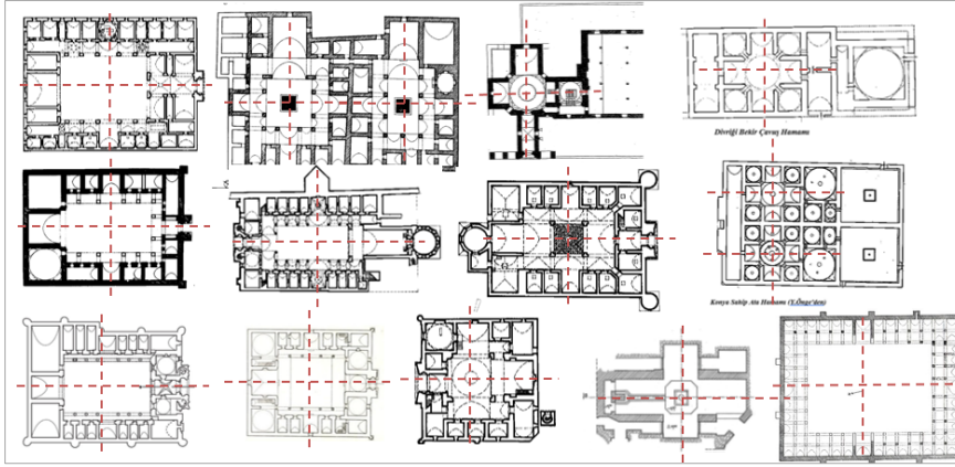
Şekil 3.5. Türk İslam Mimarlığında dört yön kurgusu (12.-13. yy)
