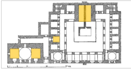
Şekil 2.112. Kasımiye Medresesi planı (Herzfeld, 1942)
