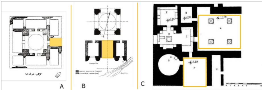
Şekil 2.28. Tureng Tepe Ateş Tapınağı (A), Gurgan Ataskuh Mahalat Tapınağı (B), (Hozhabri, 2013), Bandian Daregaz Ateş Tapınağı (C) (Tahmasbi, 2012)
