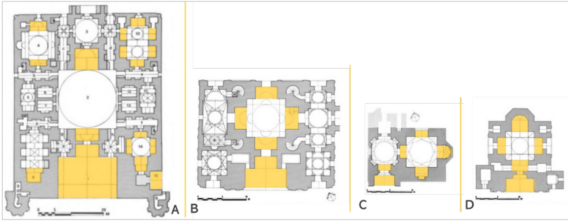
Şekil 2.126. Timurlu Dönemi Mezar Külliyesi ve Hankâhlar (A: Ahmed Yesevi Türbesi, B: Ishrat-Khaneh Türbesi, C: İsfahan Ebu Mesud Hankâhı, D: Taşkent Yunus Han Türbesi), (Golombek ve Wilber, 1988: 268, 260, 294, 267)
