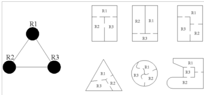
Şekil 4.1. Graf şeması ve alternatif plan şemaları (Levin, 1964)
