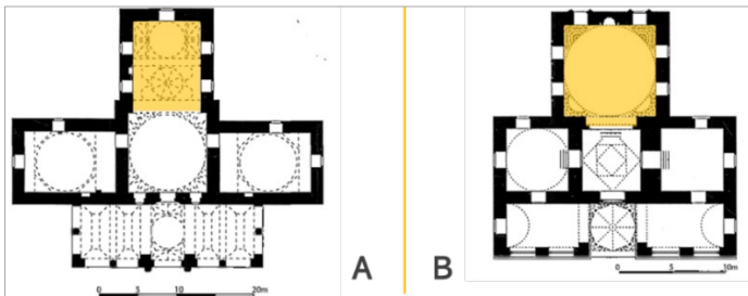
Şekil 2.103. Nilüfer Hatun İmaretî (A) ve Milas Firuz Bey İmaretî (B) planı (Kuban, 2007: 89, 95)
