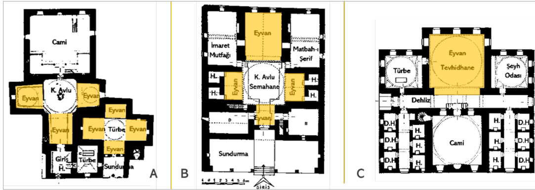
Şekil 2.114. Elvan Çelebi Zaviyesi (Eyice, 1968), Manisa Mevlevihanesi (Acun, 1992) ve Yakup Paşa Tekkesi (Tanman, 2013)
