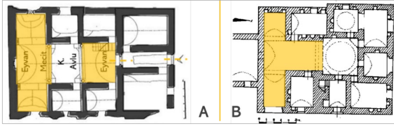
Şekil 2.82. Afyon Boyalıköy Hankâhı planı (A), (Madran, 1974), Diyarbakır Eğil Tekkesi planı (B), (Ünal, 1975)
