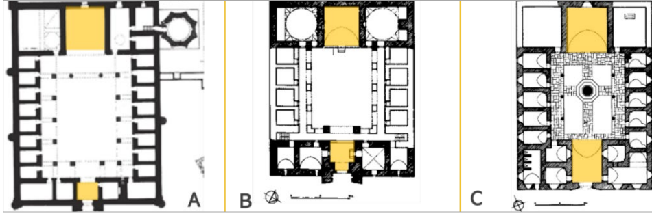
Şekil 2.71. Kayseri Hunat Hatun Medresesi, Konya Sırçalı Medrese ve Sinop Pervane Medresesi planları (Kuran, 1969: 71, 74, 86)
