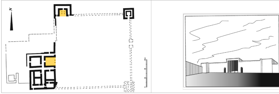
Şekil 2.15. Mansur Tepe'deki eyvanlı yapının sütunlu versiyonu (Koshelenko (КОШЕЛЕНКО) ve Gaibov (ГАЙБОВ), 2011)
