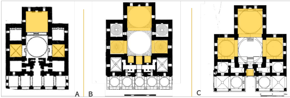
Şekil 2.104. Bursa Yıldırım (A), Yeşil (B) ve Muradiye (C) zaviyeli camilerinin planları (Kuban, 2007: 93, 98, 114)
