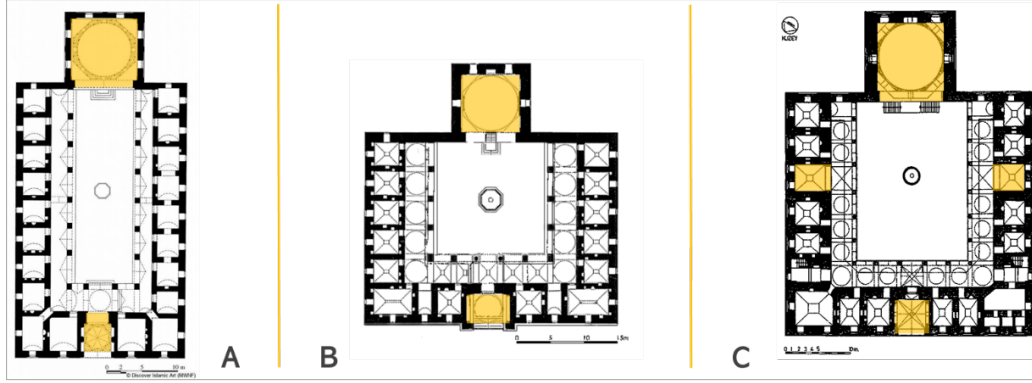
Şekil 2. 108 Bursa Yıldırım (A), Muradiye (B) ve Yeşil (C) Medreseleri planları (Kuban, 2007: 93, 97, 115)
