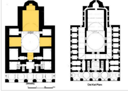
Şekil 2.102. Bursa Hüdavendigâr Camii Planı (Kuban, 2007: 86)
