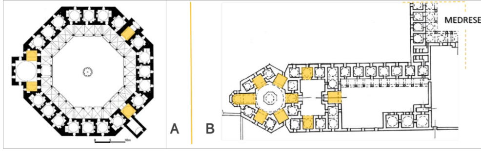
Şekil 2.111. Amasya Kapıağası Medresesi (A) ve II. Bayezid Şifahanesi (B) planları (Cantay, 2023: 273; Kuban, 2007: 221)
