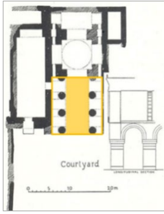
Şekil 2.27. Tepe Hisar’da bulunan kubbeli oda ve sütunlu eyvan örneği (Fontana, 2011)
