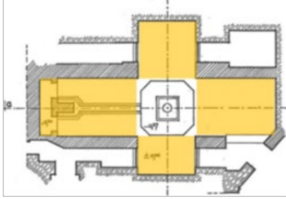
Şekil 2.86. Diyarbakır Artuklu Sarayı planı (Altun, 1977: 220)
