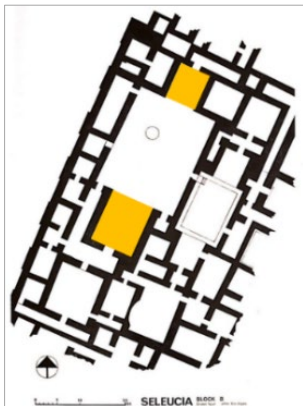
Şekil 2.5. Seleucia Tigris'te eyvanlı-avlulu konutlar (Keall, 1974)
