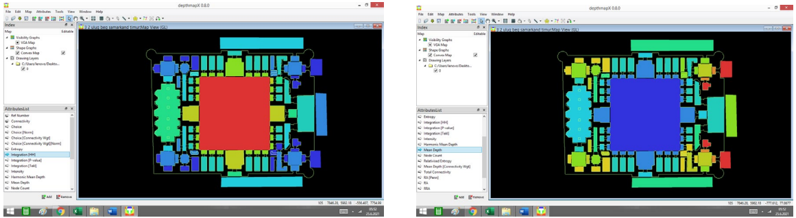
Resim 4.2. Dış bükey bütünleşme ve ortalama derinlik haritaları
