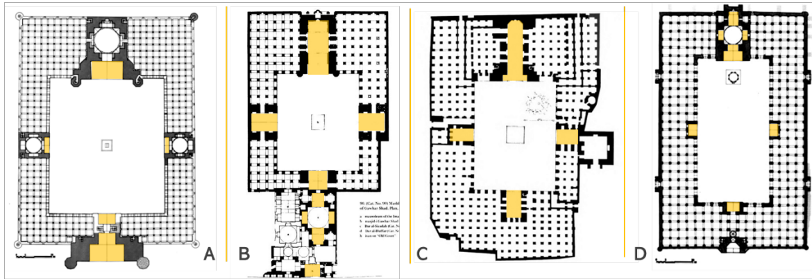
Şekil 2.124. Semerkant Bibi Hanım Camisi (A), Meşhet Gevher Şad Camisi (B), Herat Mescid-i Cuması (C) ve Buhara Kalyan Camisi (D), (Golombek ve Wilber, 1988: 255, 280, 276, 248)
