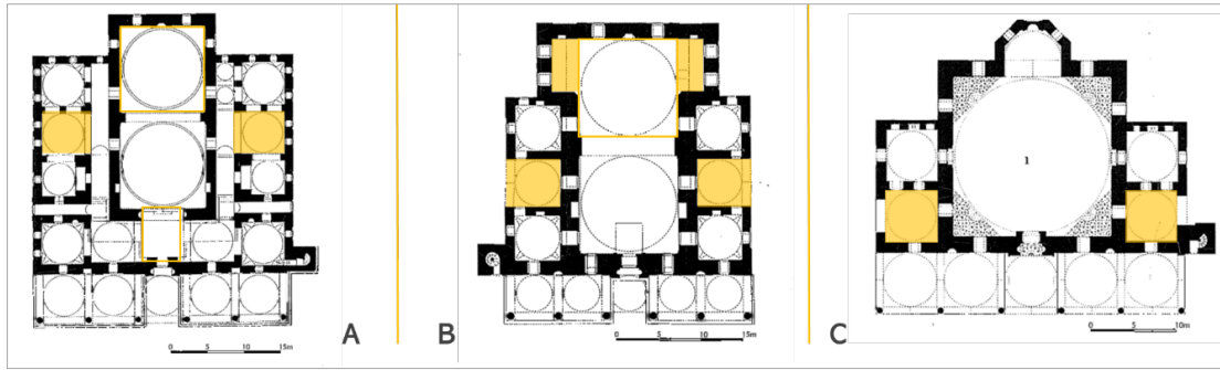
Şekil 2.106. İstanbul Mahut Paşa (A), Afyon Gedik Ahmet Paşa (B) ve İstanbul Davut Paşa (C) Camilerinin planları (Kuban, 2007: 190, 193, 211)
