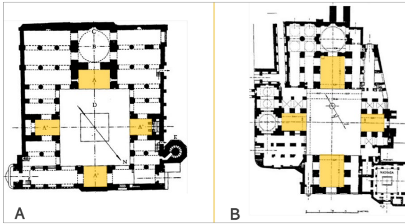
Şekil 2.57. Zevvare Mescid-i Cuması (A), Ardistan Mescid-i Cuması planı (B) (Godard, 1965: 278, 293)
