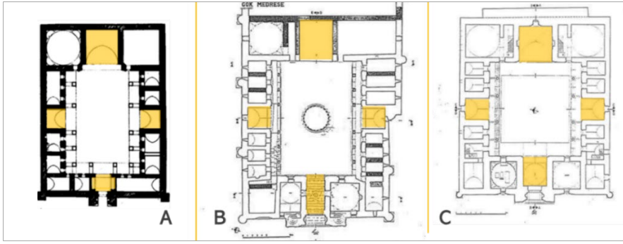
Şekil 2.72. Kayseri Sahabiye Medresesi planları (A), (Kuran, 1969: 88), Sivas Gök Medrese (B) ve Buruciye Medresesi (C) restitüsyon planı (Hersek, 2001)
