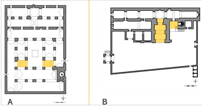
Şekil 2.65. Harput Ulu Cami (A) ve Hasankeyf Ulu Cami (B) planları (Arslan, 2017)
