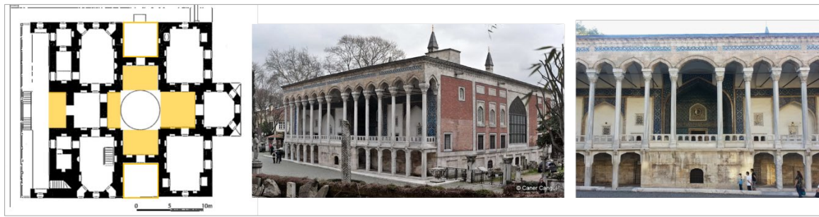
Şekil 2.117. Çinili Köşk planı (Kuban, 2007: 187), cepheler (Cangül, 2010) ve giriş eyvanı
