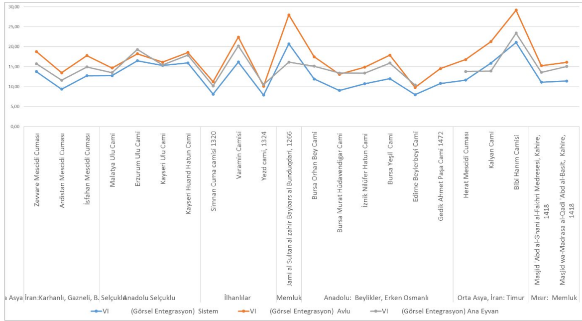
Şekil 5.3. Tüm cami örneklerine ait görsel bütünleşme değerlerinin çizgi grafiği üzerinden gösterimi
