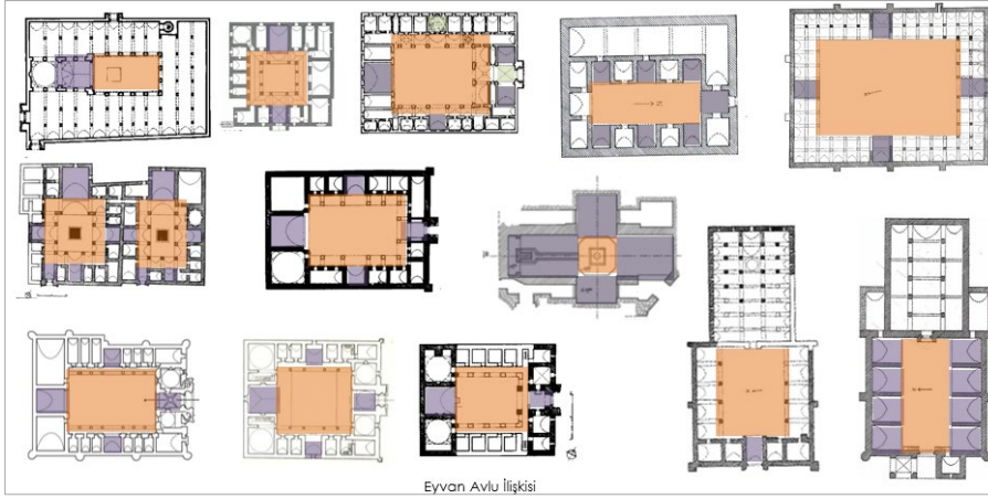
Şekil 3.8. Eyvan avlu ilişkisi (12- 13. Yy)
