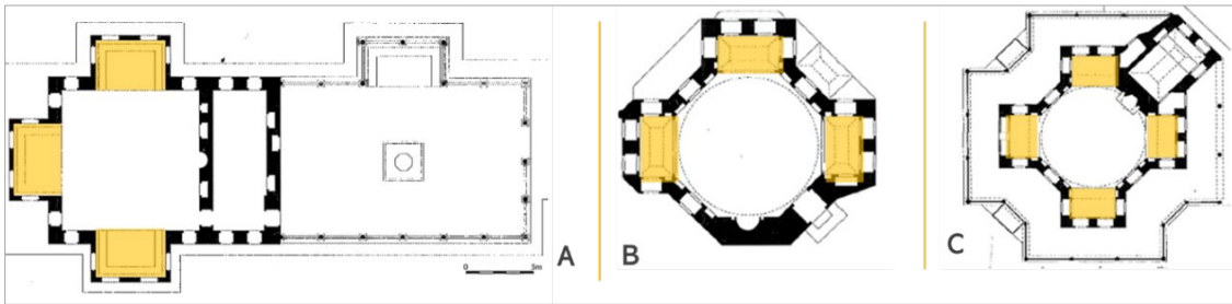
Şekil 2.133. Sepetçiler Kasrı (A), Revan (B) ve Bağdat (C) köşkleri planları (Kuban, 2007: 432, 433, 434)
