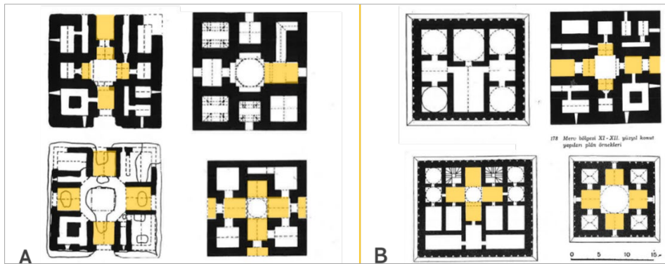
Şekil 2.48. Horasan'da Ortaçağ'da merkezi kubbeli eyvanlı konutlar, A: Tirmiz 12-13. yy konutları B: Merv 9-12. yy konutları (Cezar, 1977: 216-218)
