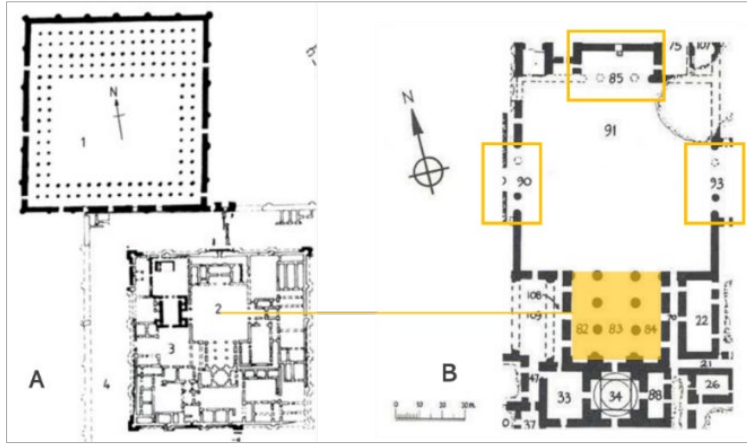
Şekil 2.43. Kûfe Dar el-İmarası A: (Nicolle, 2008: 8) B: (Fontana, 2011)
