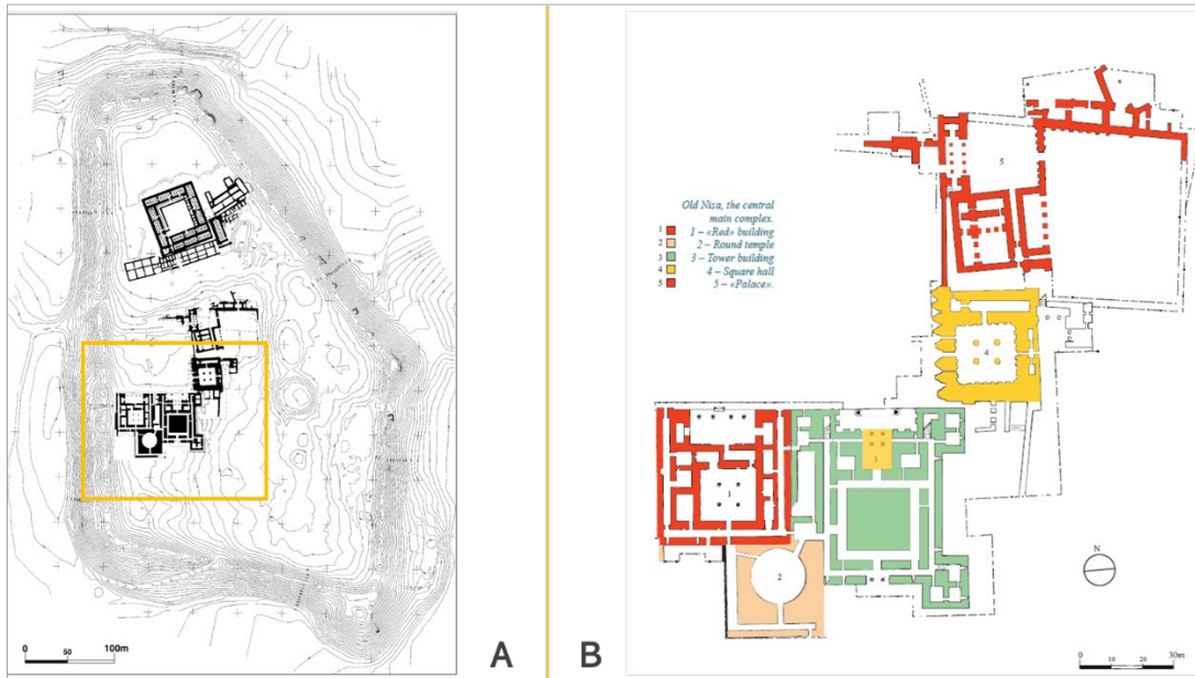
Şekil 2.16. Eski Nisa vaziyet planı (A), (Lippolis, 2006) ve Kule binası (yeşil renkli), (B), (Lippolis, 2011)
