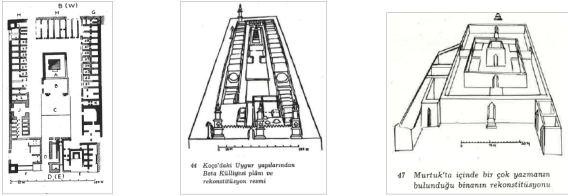
Şekil 2.35. Hoço Beta Külliyesi plan ve rekonstrüksiyonu, Murtuk A Tapınağı rekonstrüksiyonu, (Cezar, 1977: 75, 77).
