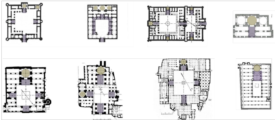
Şekil 3.13. Eyvan ve mihrap önü kubbe ilişkisi
