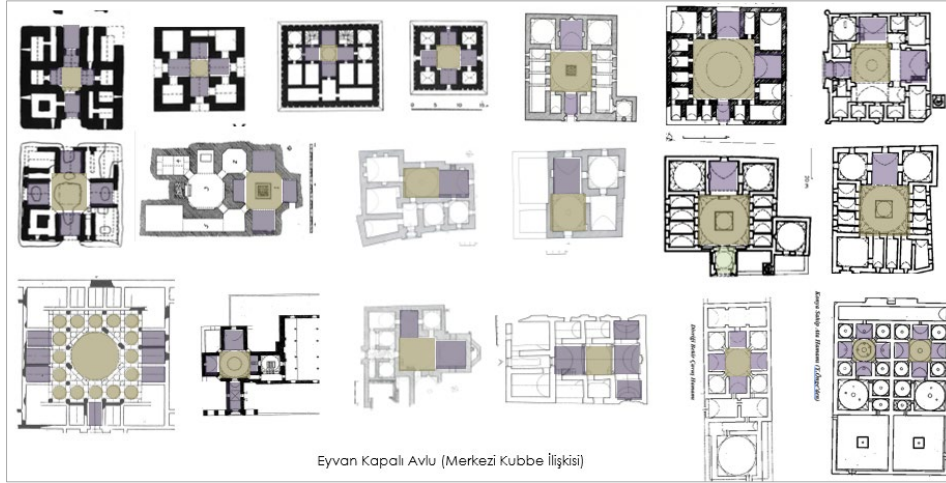
Şekil 3.9. Eyvan merkezi kubbe ilişkisi (9. – 13. Yy)
