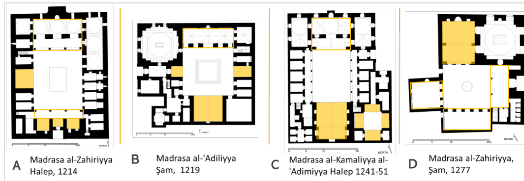
Şekil 2.91. Suriye Eyyubi dönemi medreseleri, (Planlar (Arida, 2003a, 2003b, 2003c, 2003d)
