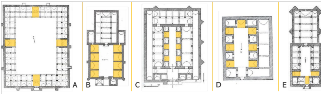
Şekil 2.88. Evdır Han (A), Kızılören Han (B), Alara Han (C), Afşin Eshab-ı Kehf Han (D), ve Ertokuş Han (E) Planları, (Erdmann, 1961: Tafel, xxix, iii, xxxii, iv)
