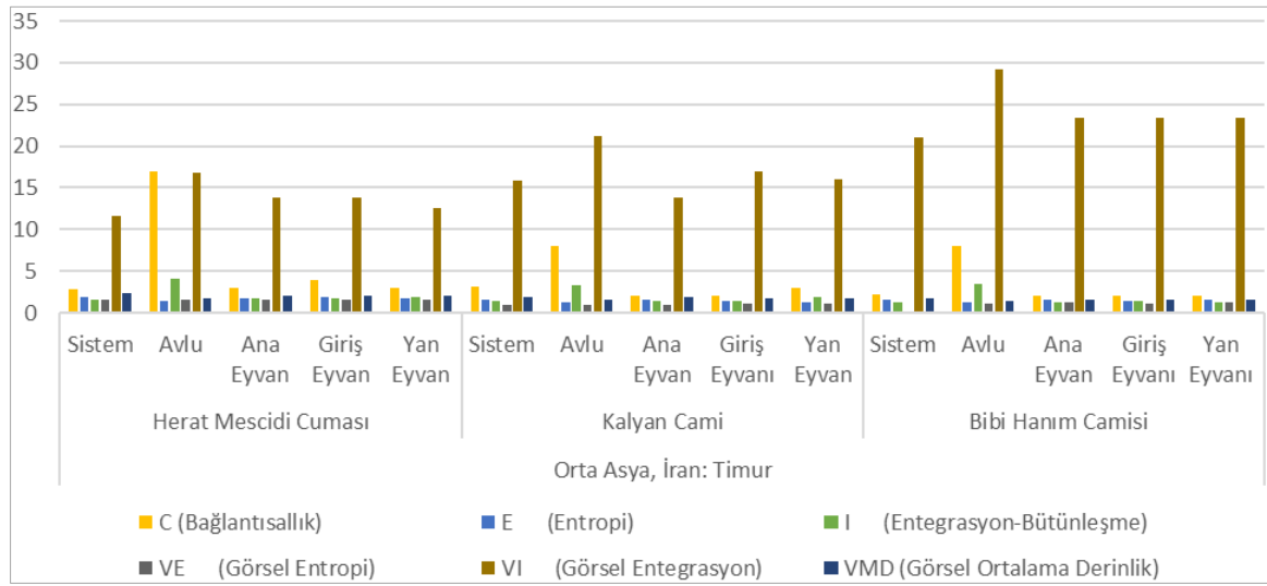
Şekil 4.21. Örneklere ait analiz verilerinin sütun grafiği
