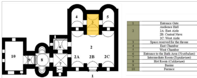
Şekil 2.38. Kusayru Amra Kasrı planı (Al-kheder, Al-shawabkeh ve Haala, 2009)
