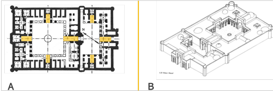
Şekil 2.63. Ribat-ı Şerif A: (Godard, 1965: 296), B: (Hillenbrand, 2000: 345)
