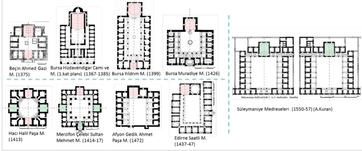
Şekil 2.113. Selçuklu sonrası medreselerde farklı kurgularda eyvan kullanımı ve Klasik Osmanlı dönemi ile eyvanın yerini kapalı dersliğe bırakması
