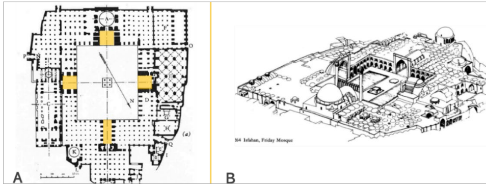
Şekil 2.59. İsfahan Mescid-i Cuması A: (Godard, 1965: 280), B: (Hillenbrand, 2000: 104)
