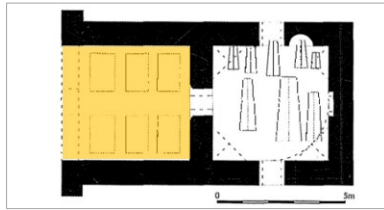
Şekil 2.115. İznik Kırğızlar (Kırk Kızlar) Türbesi planı (Kuban, 2007: 154) ve fotoğrafı (Bursa Turizm Portalı, 2023)
