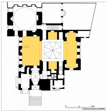
Şekil 2.122. Sultan Kayıtbay Külliyesi planı (Torky, 2023c)
