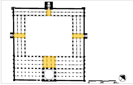
Şekil 2.94. Sultan al Zahir Baybars al Bunduqdari Cami planı (Creswell, 1978)
