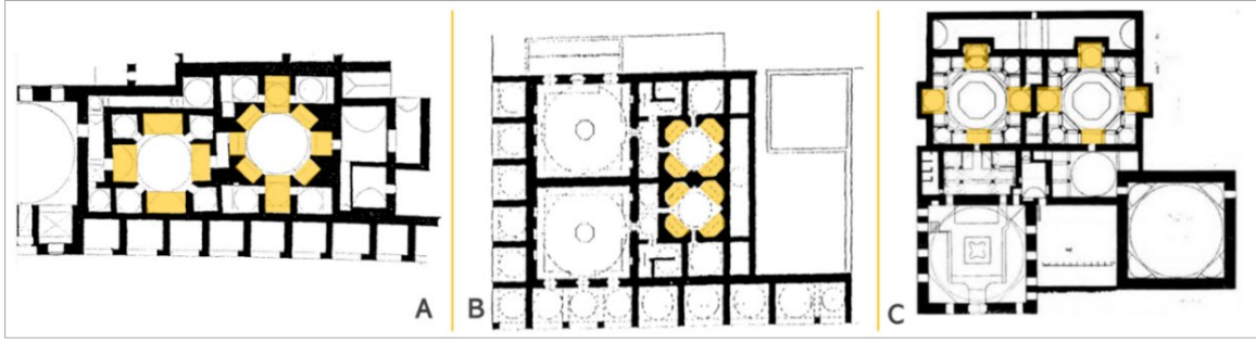
Şekil 2.131. Payas (A) ve Lüleburgaz (B) Sokullu Mehmed Paşa hamamları (Önge, 1989) ve Cağaloğlu Hamamı (Glück, 1921)
