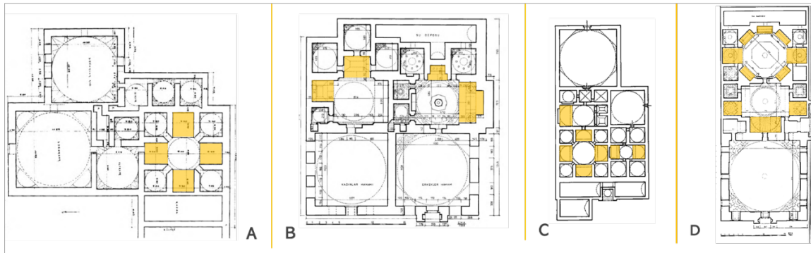
Şekil 2.116. Bursa Orhan Gazi Hamam ve Bursa’daki Mahkeme Hamamı Planı (E. H. Ayverdi ve Yüksel, 1976: 108-109), Edirne Tahtakale hamamı Planı (Akçıl, 2010), İstanbul Mahmud Paşa Hamamı (E. H. Ayverdi ve Yüksel, 1976: 112)
