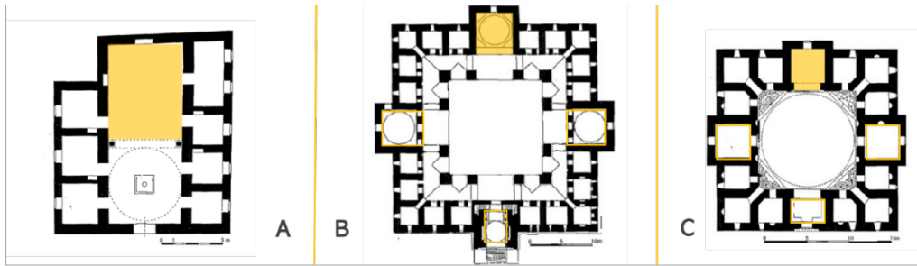
Şekil 2.109. Bursa Lala Şahin Paşa (A), Merzifon Çelebi Sultan Mehmet (B) ve Gümüş Hacı Halil Paşa (C) Medreseleri (Kuban, 2007: 150, 152)
