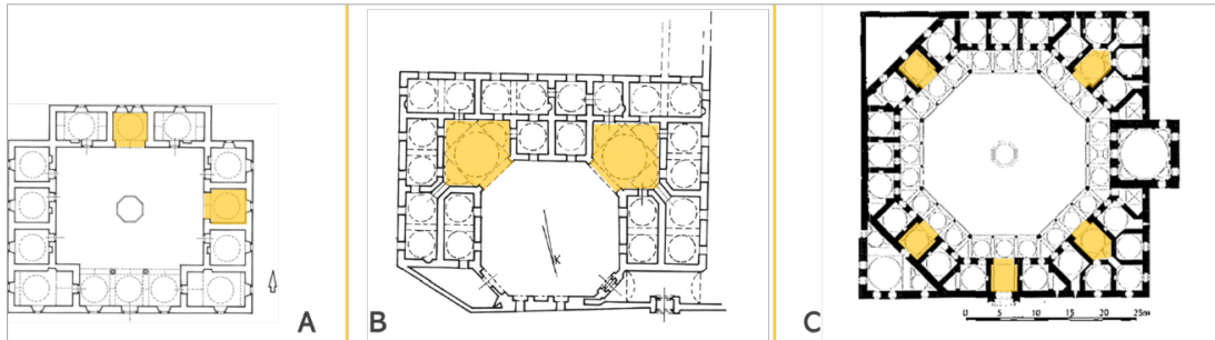
Şekil 2.129. Manisa Hafsa Sultan (A) ve İstanbul Haseki (B) Şifahaneleri (Cantay, 2023: 257, 273), İstanbul Rüstem Paşa Medresesi (C) (Kuban, 2007: 221) planları
