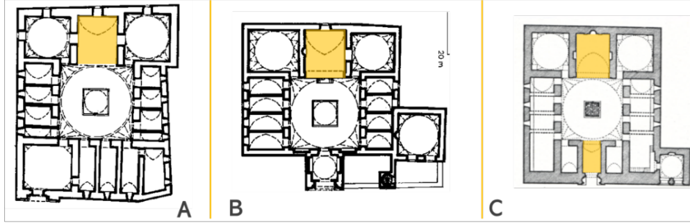
Şekil 2.69. Konya Karatay Medresesi (A) ve İnce Minareli Medrese planı (B), (Schneider, 2000), Afyon Çay Taş Medrese planı (C), (Kuran, 1969: 58)
