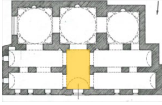
Şekil 2.64. Siirt Ulu Cami planı (Aslanapa, 1989: 104)
