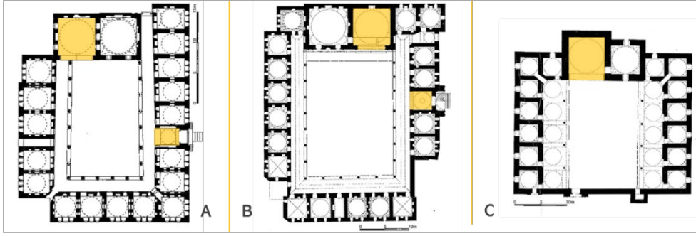
Şekil 2.110. Edirne Saatli (A) ve Peykler Medreseleri (B) ile Afyon Gedik Ahmet Paşa Medresesi (C) Planları (Kuban, 2007: 152, 220, 194)
