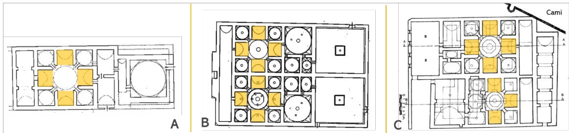
Şekil 2.87. Divriği Bekir Çavuş Hamamı (A), Sahip Ata Hamamı (B) ve Hunat Hatun Hamamı (C) planları (Karpuz, 2001: 109–110)
