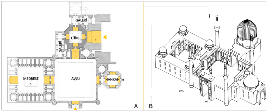
Şekil 2.127. Semerkant Gur-i Emir Külliyesi (A: plan, (Golombek ve Wilber, 1988: 256), B: Perspektif, (Hillenbrand, 2000: 300))
