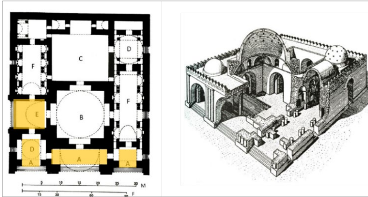
Şekil 2.23. Sarvistan Sarayı plan ve rekonstrüksiyonu (Pope, 1965a) (A: Üçlü Eyvan, B: Merkezi Kubbeli Salon, C: Avlu, D: Küçük Kubbeli Salon, E: Güney Girişi Eyvanı, F: Tonoz Örtülü Mekânlar)
