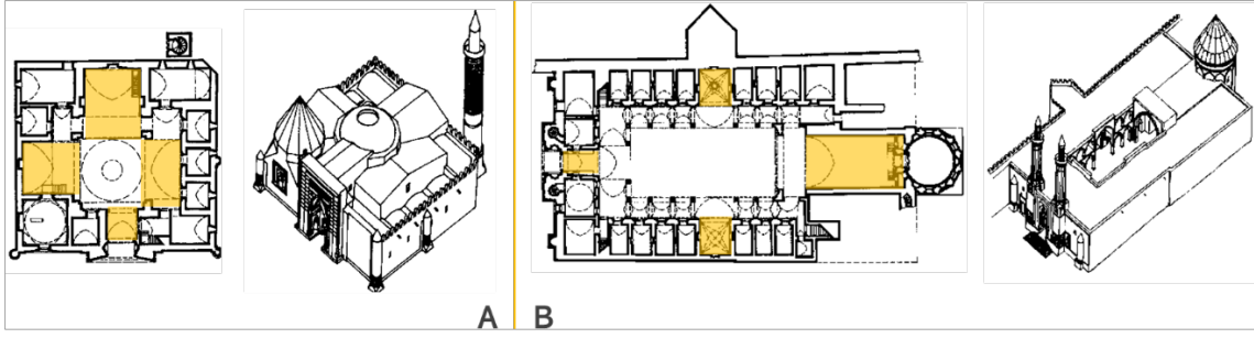
Şekil 2.75. Kırşehir Cacabey Medresesi (A) ve Erzurum Çifte Minareli Medrese (B) (Schneider, 2000)
