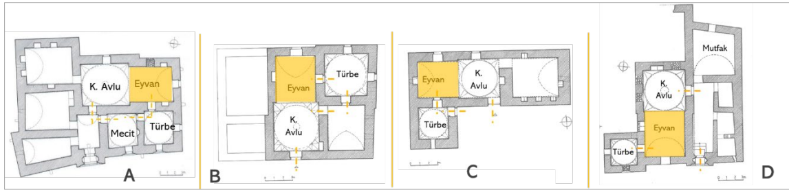
Şekil 2.80. Tokat Halef Gazi Hankâhı, Ebu's Şems Hankâhı, Şeyh Mecnun Zaviyesi, Hoca Sünbül Baba Zaviyesi Planları (Parlak, 2005)
