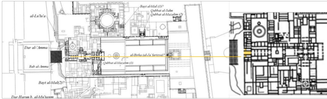
Şekil 2.41. Hakan Sarayı (el-Cevsaku'I Hakani) kısmi planı (Saba, 2015)
