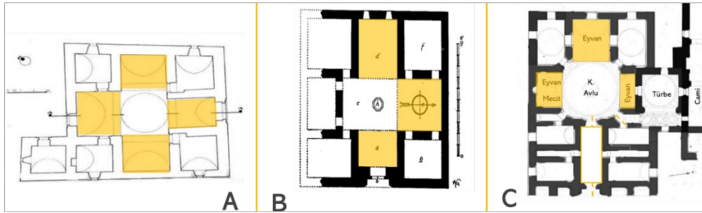
Şekil 2.81. Kayseri Ahi Evran Zaviyesi (A), Niksar Çöregibüyük Tekkesi (B), (Karpuz, 2013) ve Konya Sahip Ata Hankâhı (C), (Önge, 1984)
