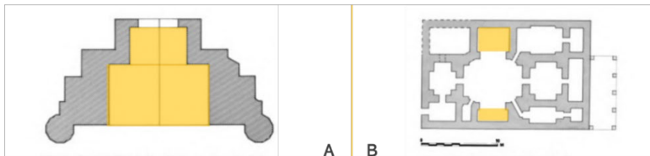
Şekil 2.128. Şehr-i Sebz Ak Saray eyvan planı (A), Şehr-i Sebz'de yer alan bir hamam planı (Golombek ve Wilber, 1988: 263, 264)
