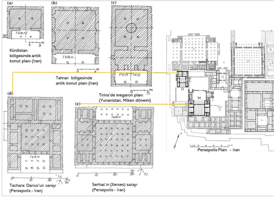
Şekil 2.8. Planlar Tavassoli'den (2020: 8) alınarak düzenlenmiştir
