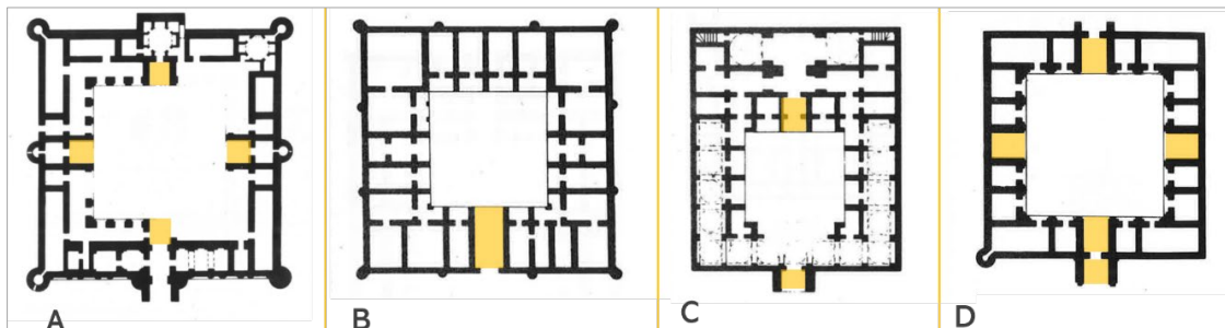
Şekil 2.54. Daya Hatun (A), Dehistan (B), El Asker (C) ve Ode Merguen (D) Kervansarayları (Cezar, 1977: 193, 195)
