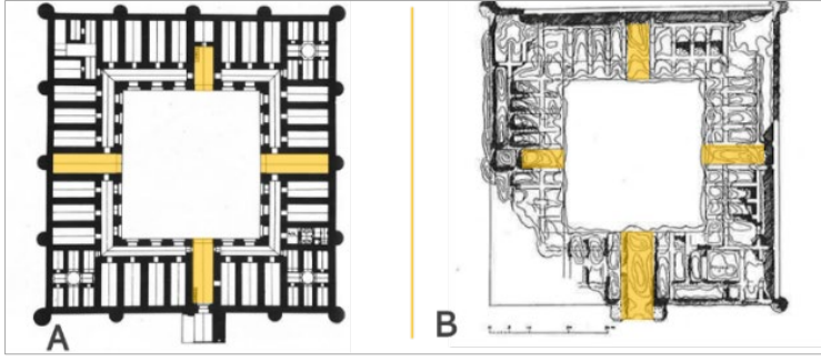
Şekil 2.62. Ribat-ı Anuşirvan ve Ribat-ı Zafarani planları (Cezar, 1977: 208-209)
