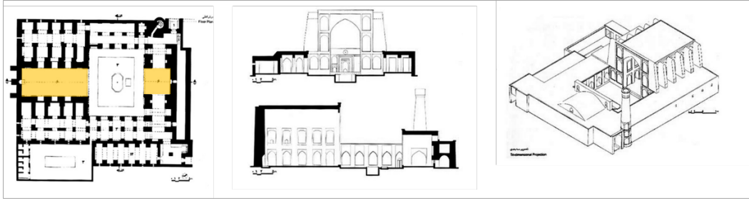
Şekil 2.46. Neyriz Cuma Camisi (Sokhanpardaz, 2020)
