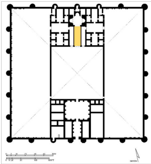
Şekil 2.39. Mişatta Sarayı planı (URL-5)
