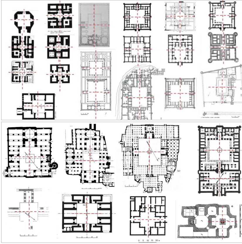
Şekil 3.4. Türk İslam Mimarlığında dört yön kurgusu (9.-11.yy)
