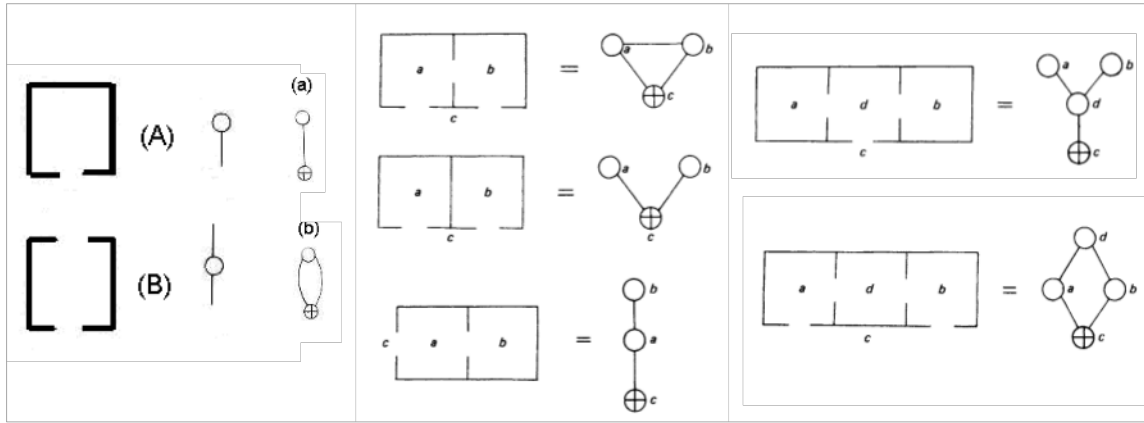
Şekil 4.2. Erişim grafikleri ile farklı mekân konfigürasyonları (Hillier ve Hanson, 1984)
