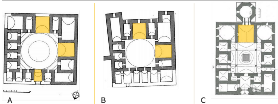
Şekil 2.68. Tokat (A) ve Niksar (B) Yağıbasan Medreseleri, Isparta Atabey Ertokuş Medresesi (C) planı (Kuran, 1969:15, 17, 48)
