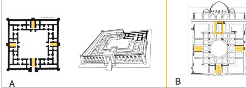
Şekil 2.53. Manakeldi Kervansarayı plan ve rekonstrüksiyonu (A), (Cezar, 1977: 186-187), Ribat-ı Melik (B), (Aslanapa, 1989: 40)
