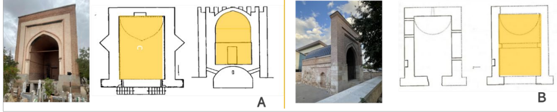
Şekil 2.77. Gömeç Hatun Türbesi (A) ve Bedrettin Gevhertaş Türbesi (B) planlar: (Önkal, 1996: 305-342)
