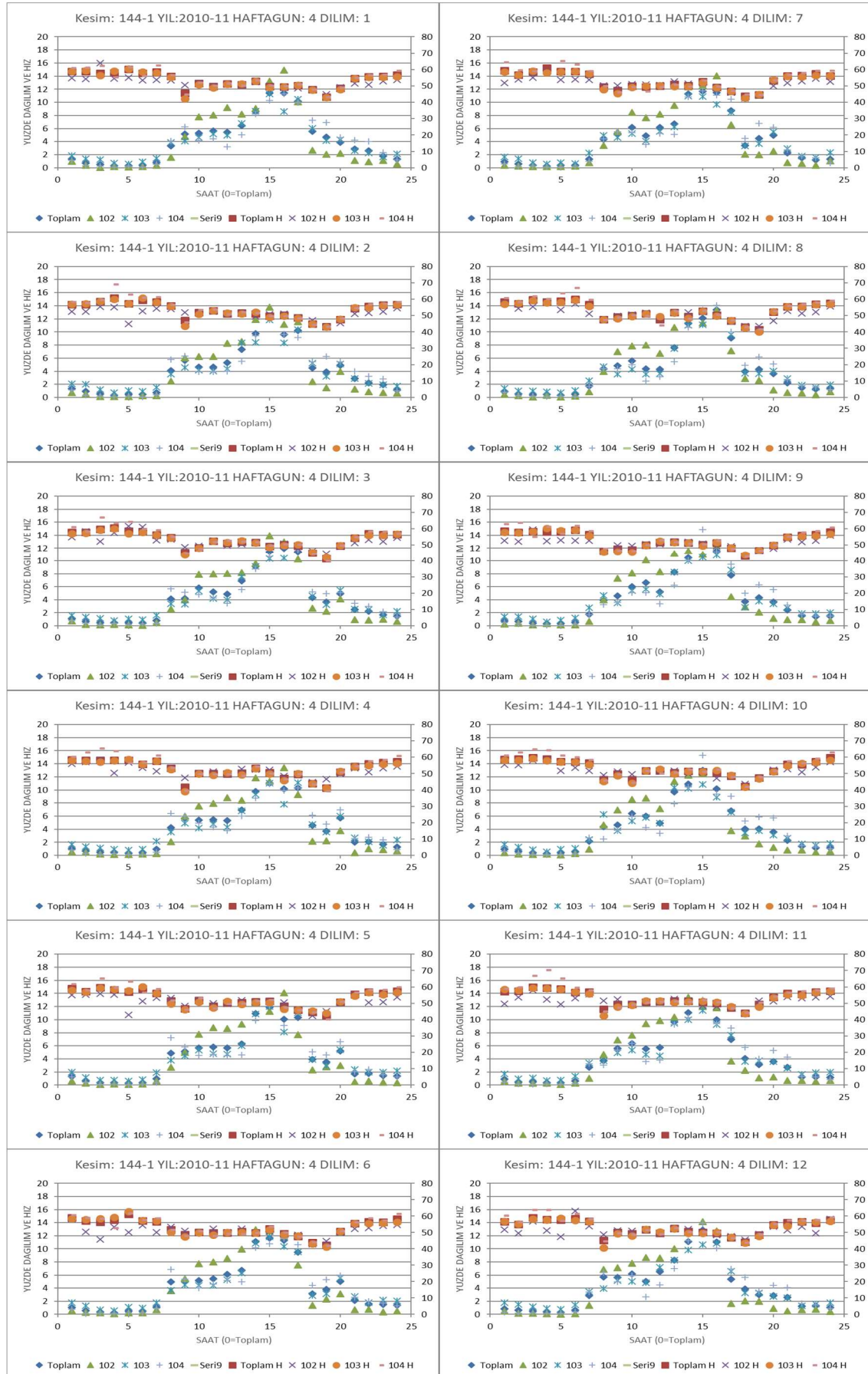
Şekil 4.33. Kesim 144; Haftağün 4 için saatlere göre dilim trafik dağılımı ve hızları
