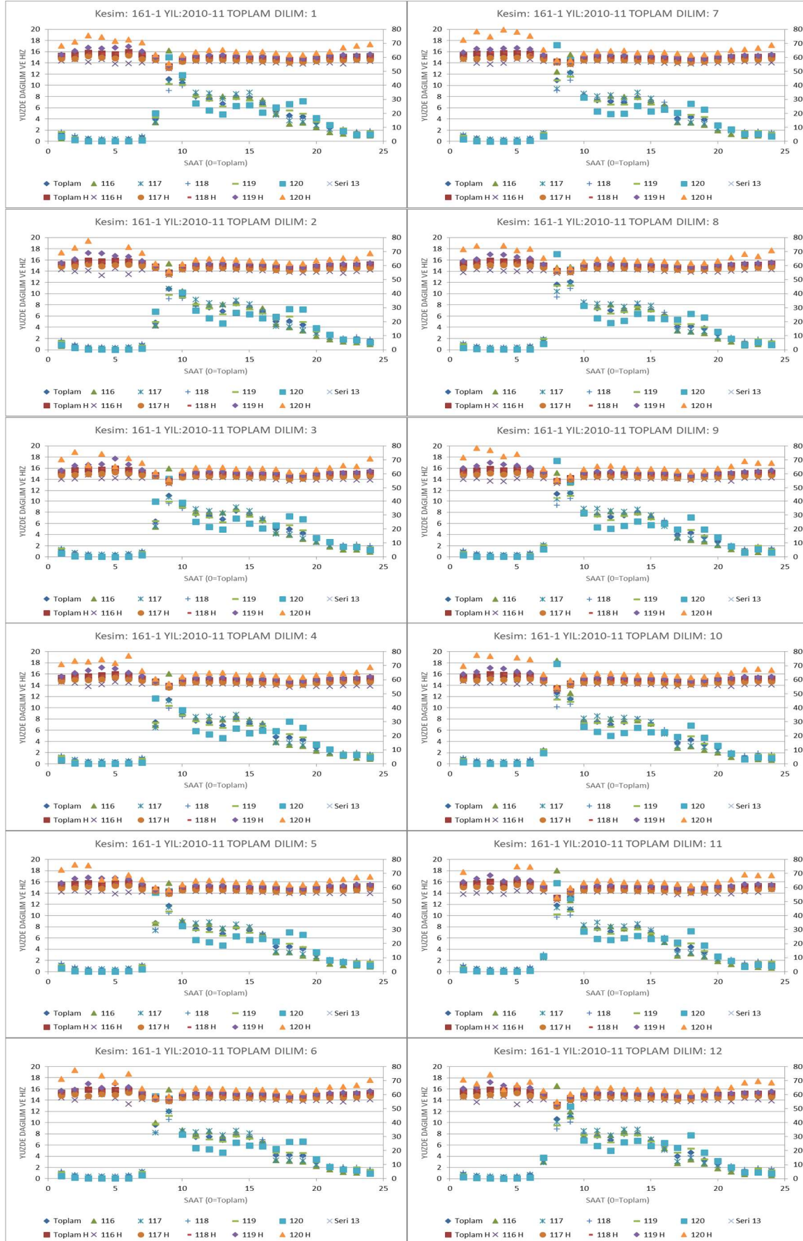
Şekil 4.49. Kesim 161; Saatlara göre toplam dilim trafik dağılımı ve hızları
