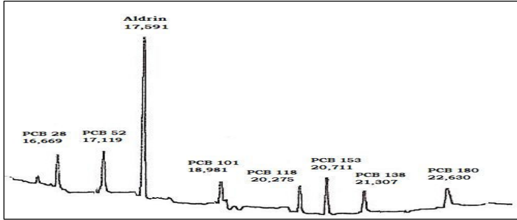
Şekil 38: 98 no'lu bireye ait örnek kromotogram
