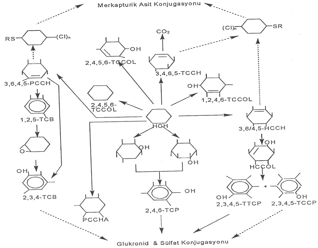
Şekil 11: Benzenheksaklorür'ün metabolizması
