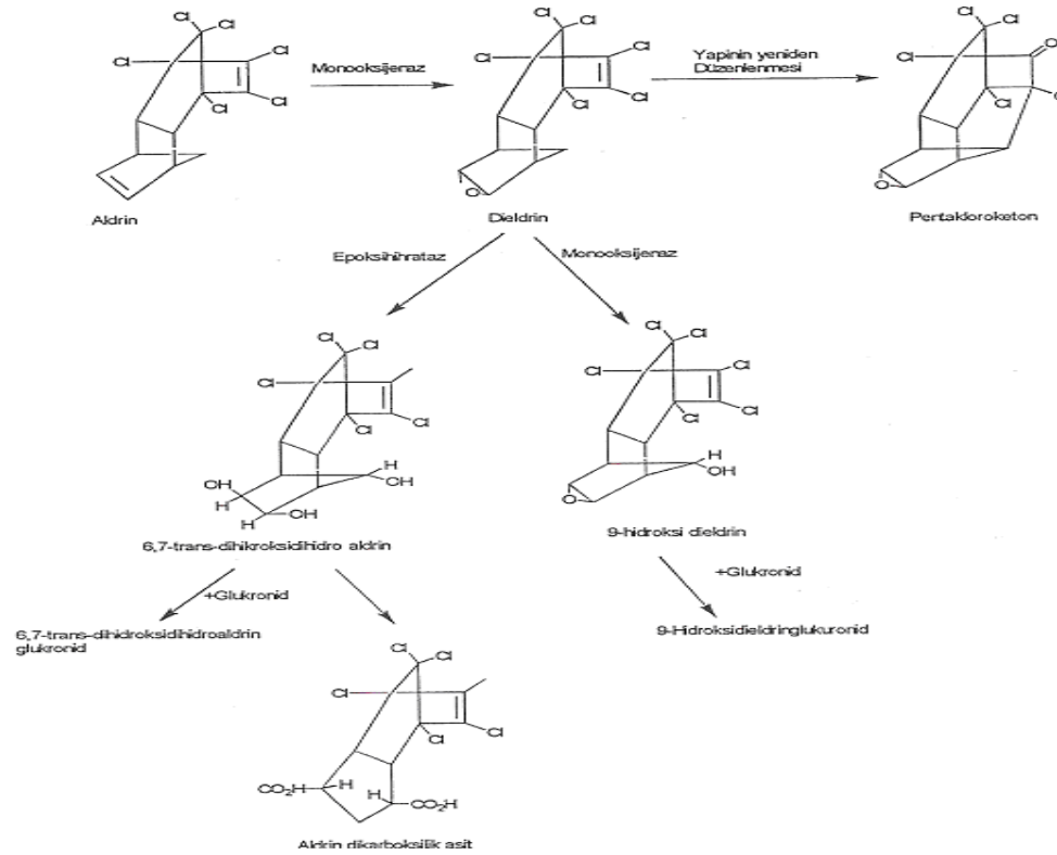
Şekil 16: Aldrin'in metabolizması
