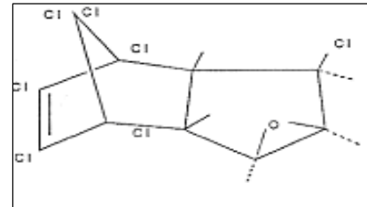
Şekil 6: Heptaklor Epoksit
