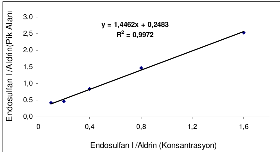
Şekil 26: \alpha -Endosülfan'ın Gaz-sıvı Kromatografisi-ECD'deki kalibrasyon eğrisi
