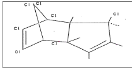
Şekil 5: Heptaklor
