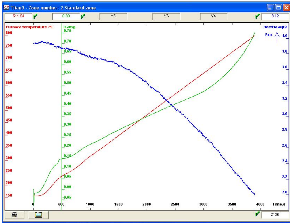
Şekil 3.1. Deneyde kullanılan Ti-Fe alaşımlarının TGA grafiği
