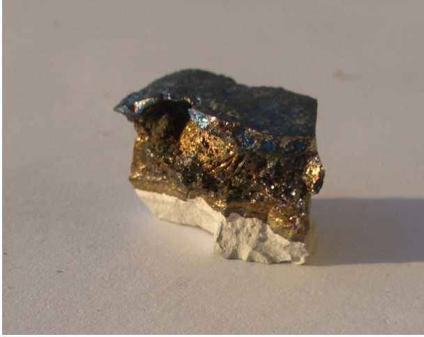
Resim 4.5. %99'luk Ar gazı beslenerek inert hale getirilmiş fırında 1600°C'de 2 saat süre bekletilen alaşım üzerindeki oksit tabakası
