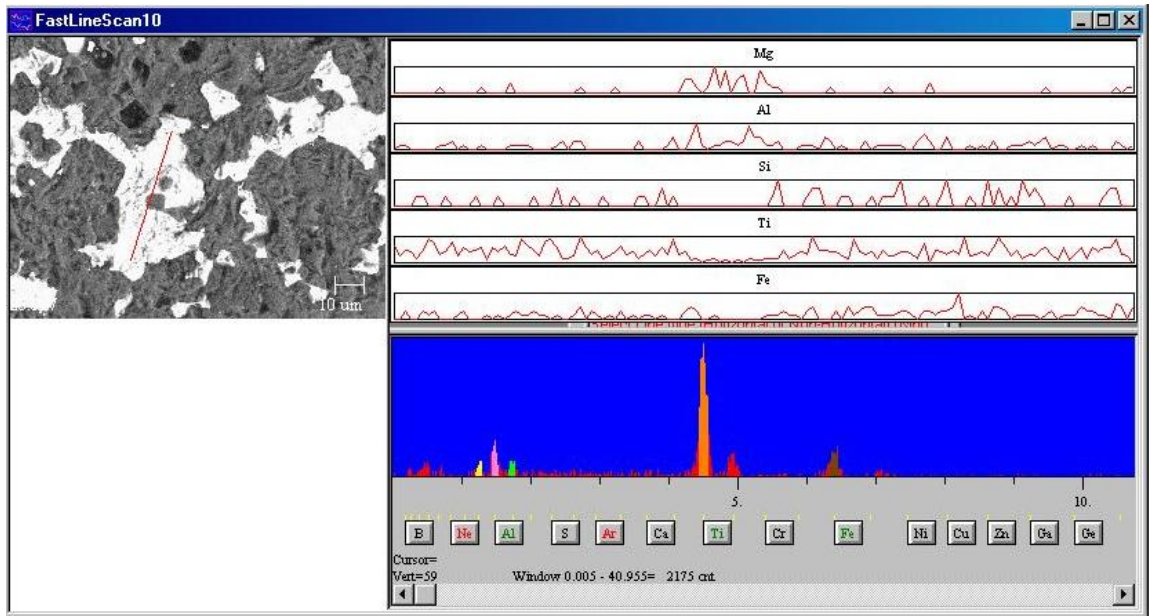
Şekil 4.6. %10 SA içeren spinel oksit malzemede EDS analizi grafiği
