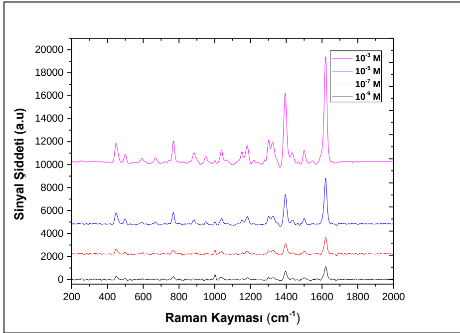
Şekil 4.33. Katlanmış iki kollu polimerik platformlarda farklı derişimlerdeki metilen mavisinden toplanan SERS spektrumları
