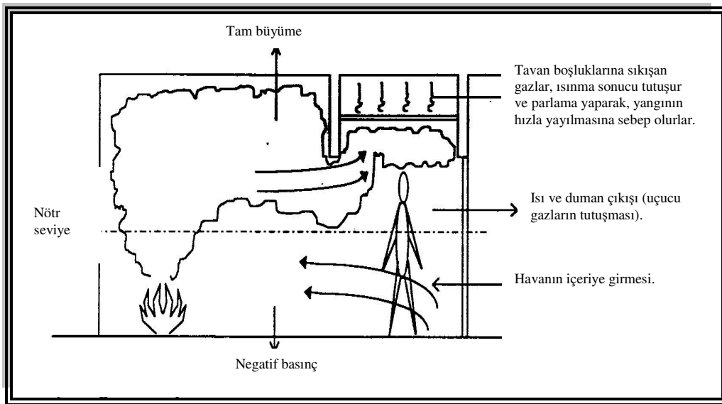
Şekil 2.4. Yangının gelişmesi [15]
