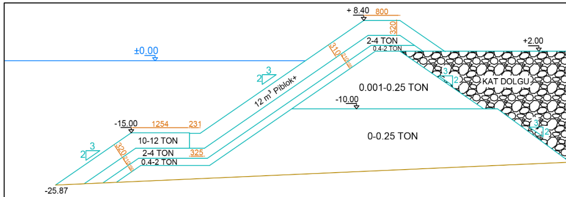
Şekil 6.42. HAD analizi yapılan Piblok+ kesiti
