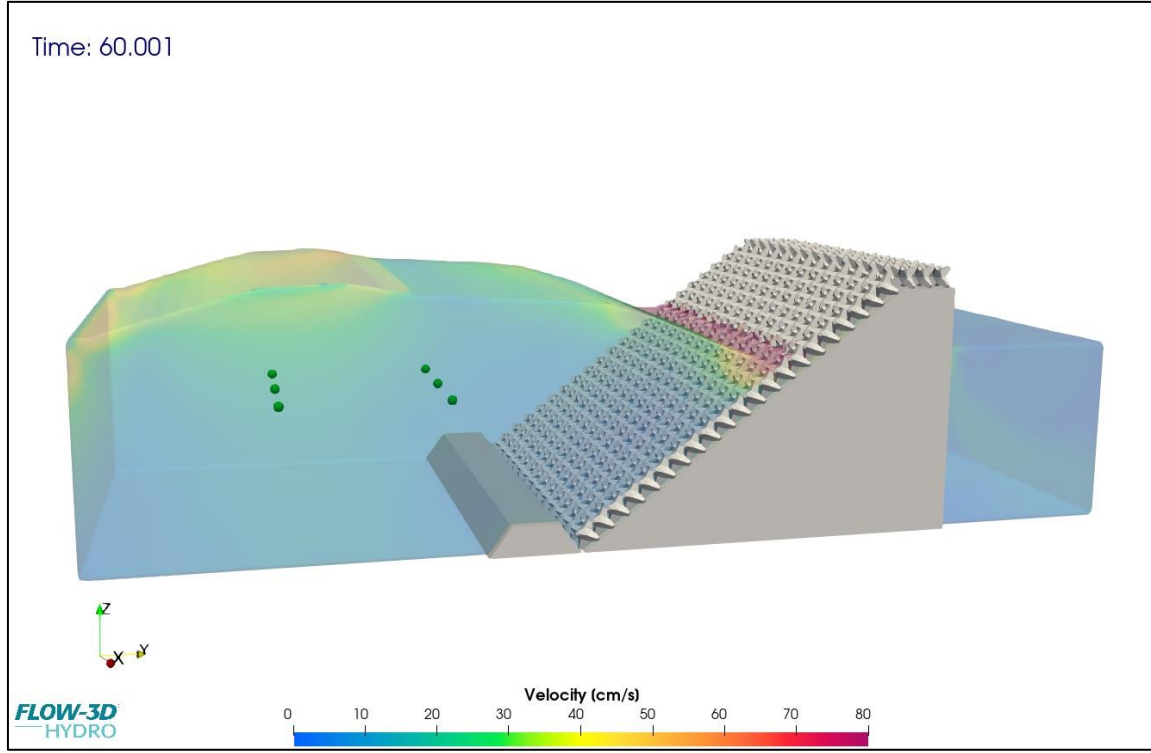
Şekil 6.27. Model bünyesinde elde edilen su partikül hızları (cm/s).
