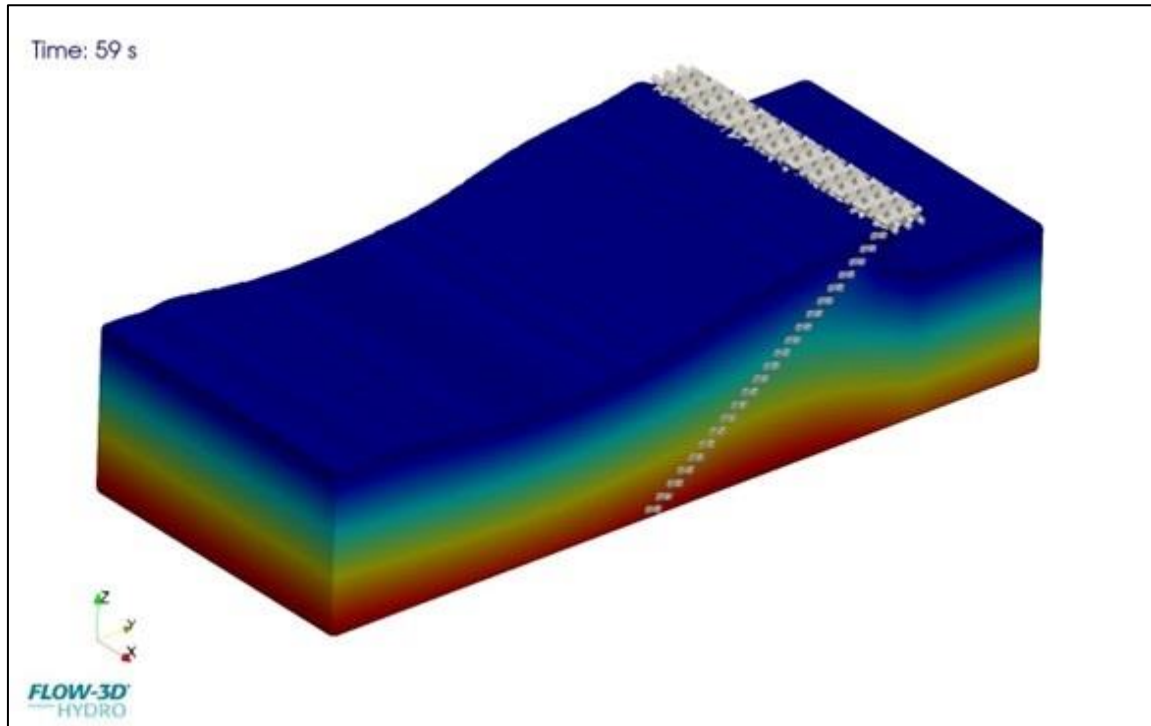
Şekil 6.36. Model bünyesinde elde edilen dalga tırmanma görseli
