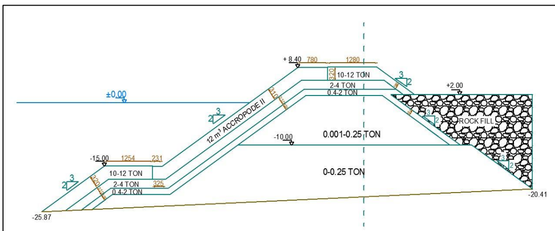
Şekil 6.41. Hidrolik model deneyleri yapılan Accropode II kesiti (Alternatif 3)
