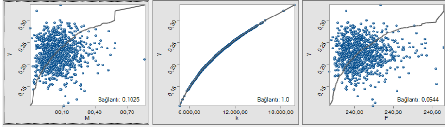
Ek-1. Şekil.6. MCS yöntemine girışı yapılan değişkenlerin saçılım grafikleri
