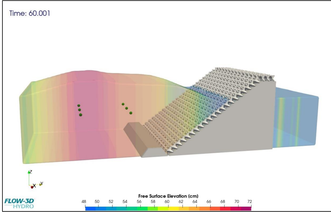
Şekil 6.25. Model bünyesinde elde edilen serbest yüzey değışimi (cm).
