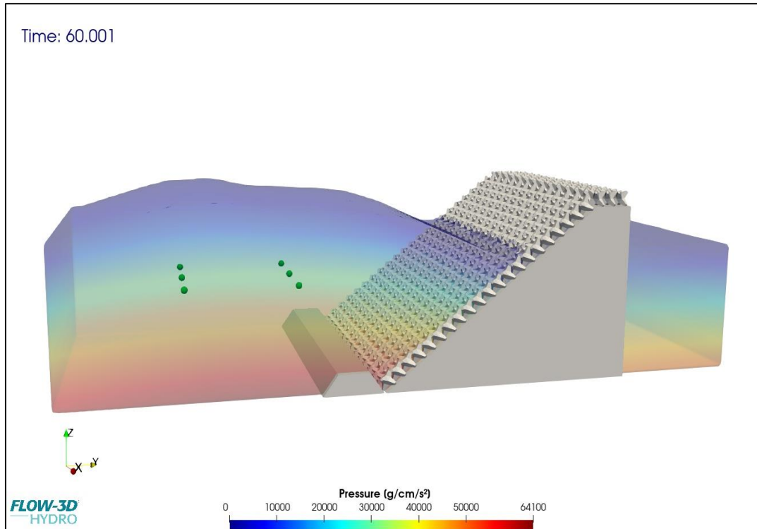
Şekil 6.26. Model bünyesinde elde edilen basınç değeri (g/cm/s²).
