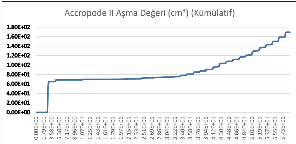
Şekil 6.38. FLOW-3D analiz sonucu elde edilen Accropode II aşma (kümülatif) değeri (cm³)
