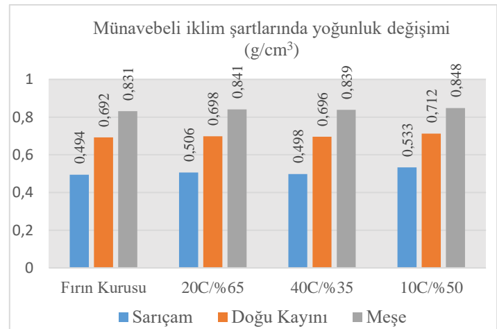
Şekil 8. Ardışık elde edilmiş yoğunluk değerleri
