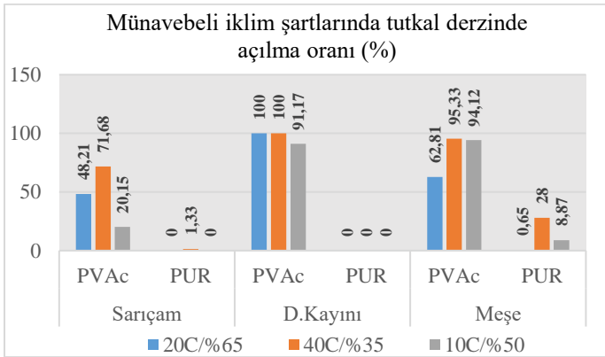
Şekil 10. Ardışık elde edilmiş delaminasyon değerleri
