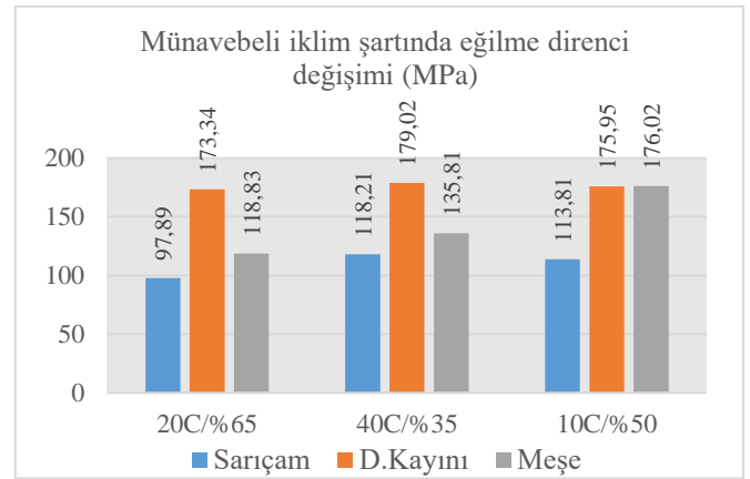
Şekil 11. Ardışık elde edilmiş eğilme direnci değerleri
