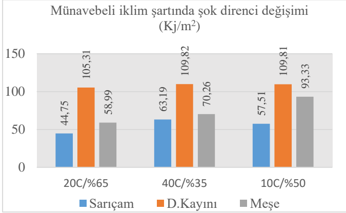
Şekil 13. Ardışık elde edilmiş şok direnci değışimleri
