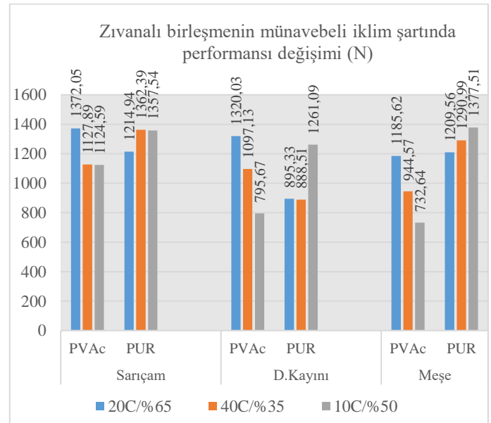
Şekil 16. Ardışık elde edilmiş zıvanalı birleşme performansı değışimleri
