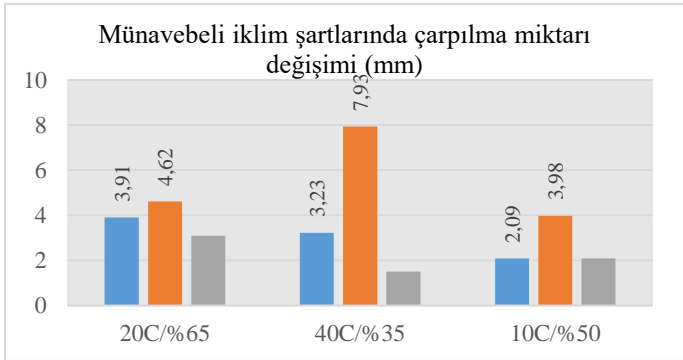
Şekil 9. Ardışık elde edilmiş çarpılma değerleri
