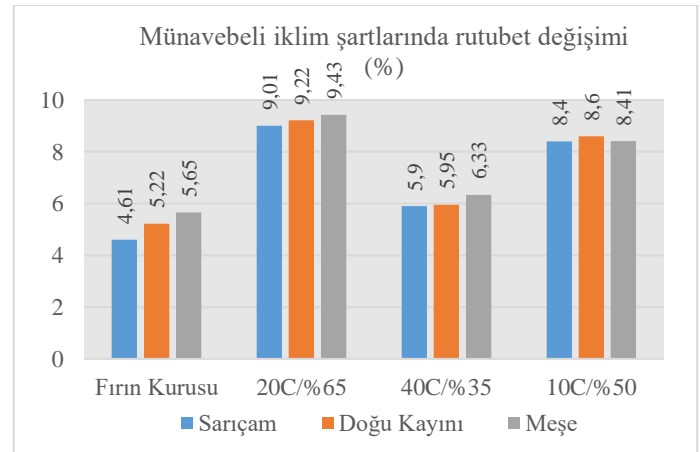
Şekil 7. Ardışık elde edilmiş denge rutubeti değerleri
