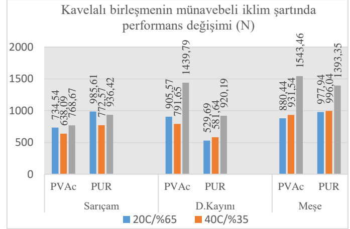
Şekil 15. Ardışık elde edilmiş kavelalı birleşme performansı değışimleri
