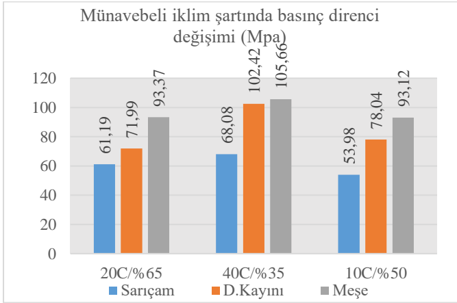
Şekil 14. Ardışık elde edilmiş basınç direnci değışimleri
