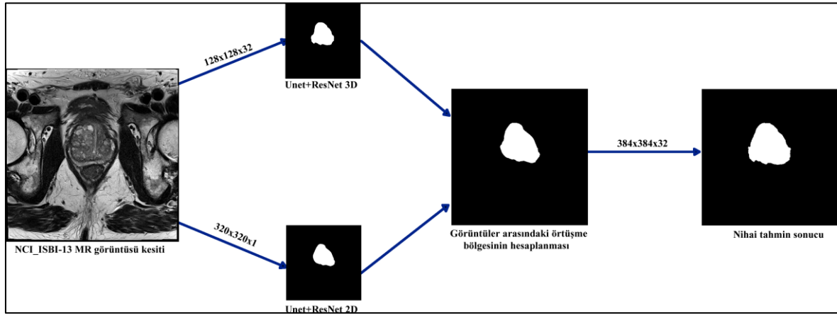
Şekil 5. 3. Önerilen füzyon modelin NCI_ISBI-13 veri seti üzerindeki bölütleme aşamaları
