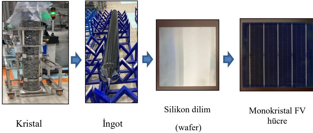
Şekil 3.2. Monokristal FV hücre ve temel üretim aşamaları
