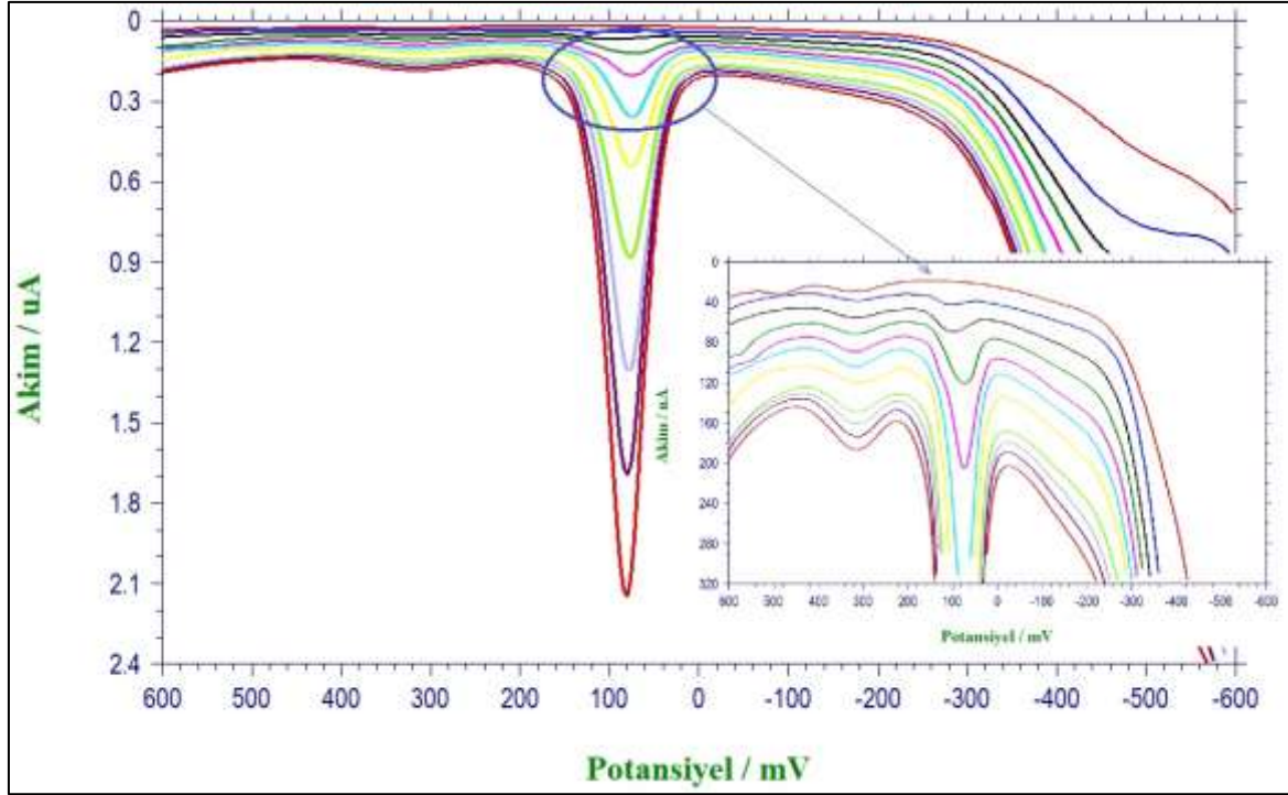
Şekil 5.10. 10 mL pH=7,0 fosfat tamponu içerisinde 3,38 \times 10^{-6} M'dan 1,84 \times 10^{-5} M'a kadar \text{Hg}^{2+} 'nin anodik yönde kare dalga voltametri ile alınan voltamogramları
