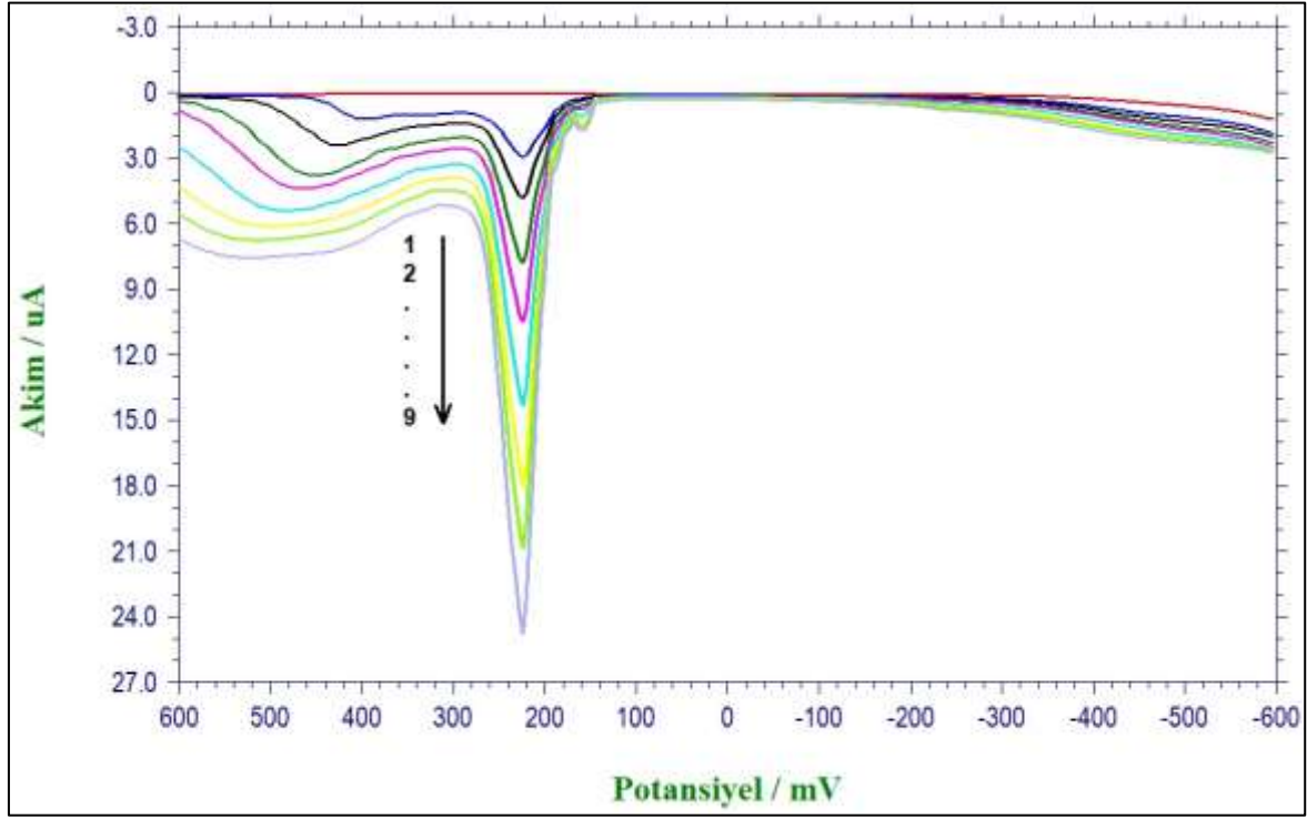
Şekil 5.12. Kare dalga voltametri ile 1,0 \times 10^{-2} M standart \text{Hg}^{2+} iyonu ile yapılan kalibrasyon grafiği çalışması
