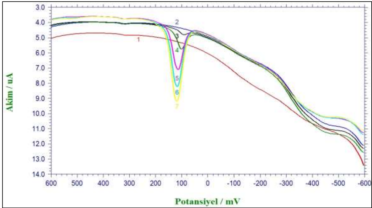
Şekil 5.20. Sentetik örnekteki 4,85 \mu\text{M} civa(II)'nin anodik kare dalga voltametrisi kullanılarak standart ekleme metodu ile tayini
