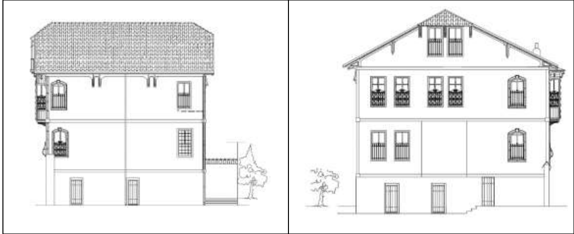
Resim 5.167. Takkasızlar Konağı batı ve güney cephesi (Gonca AYDIN ADALI arşivinden yararlanılarak yeniden çizilmiştir)
