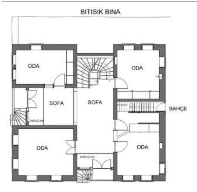
Resim 5.157. Takkasızlar Konağı zemin kat planı (Gonca AYDIN ADALI arşivinden yararlanılarak yeniden çizilmiştir)
