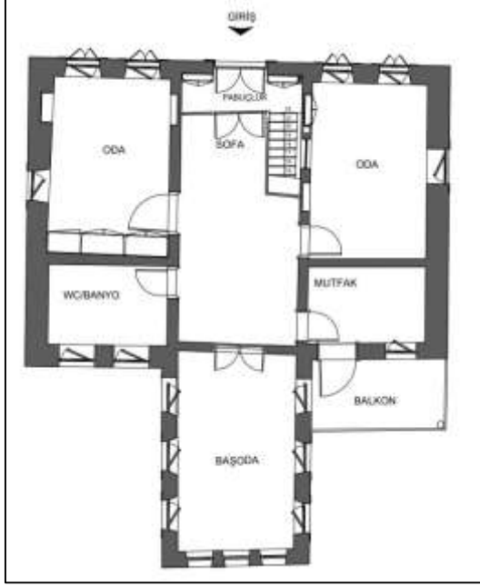
Resim 5.94. Tuncer Öz (Papazın Evi) zemin kat planı (Mustafa Korumaz Arşivi, 2016)
