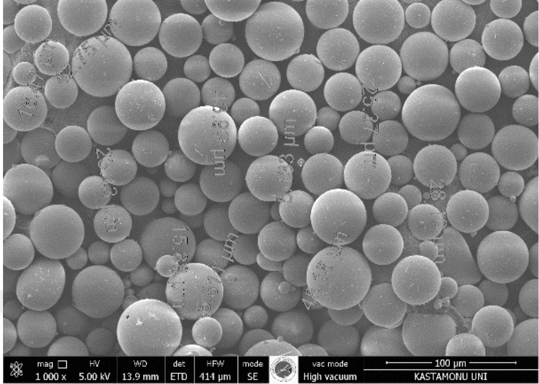
Şekil 3.7 Seramik küreciğin 1000 kat büyütülmüş SEM görüntüsü
