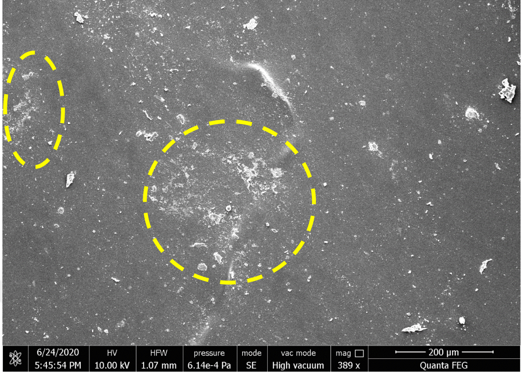
Şekil 5.7 D99 vernik katmanında ZnO'in 1 nolu SEM görüntüsü
