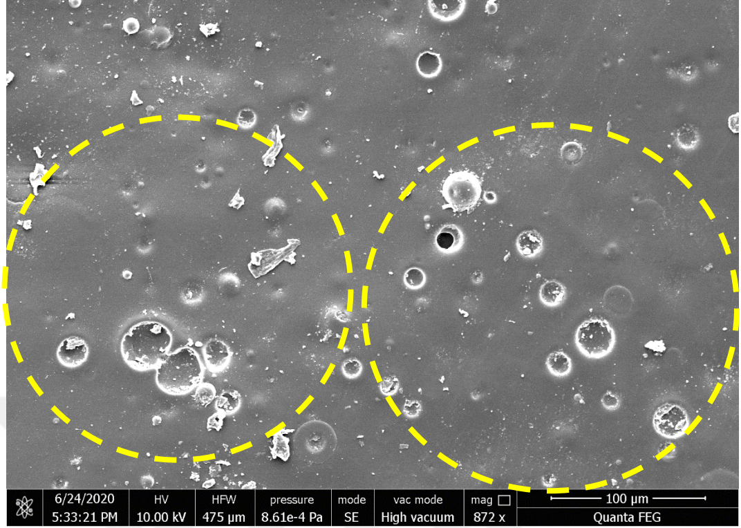
Şekil 5.5 D70 vernik katmanında seramik küreciğın SEM görüntüsü
