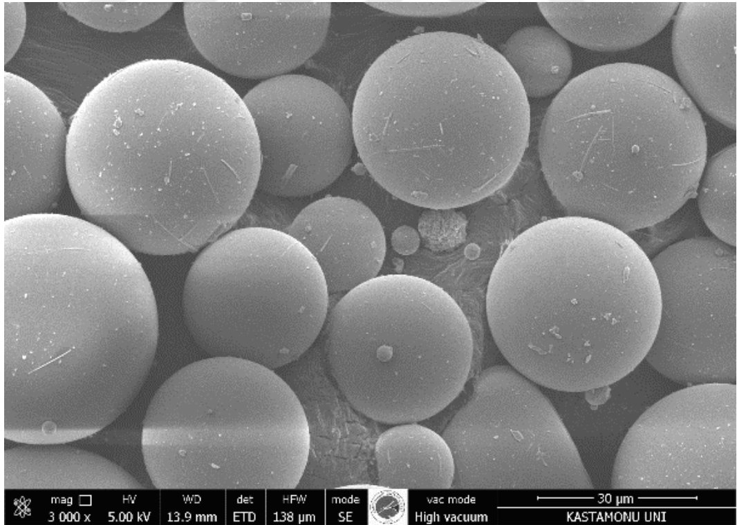
Şekil 3.8 Seramik küreciğin 3000 kat büyütülmüş SEM görüntüsü
