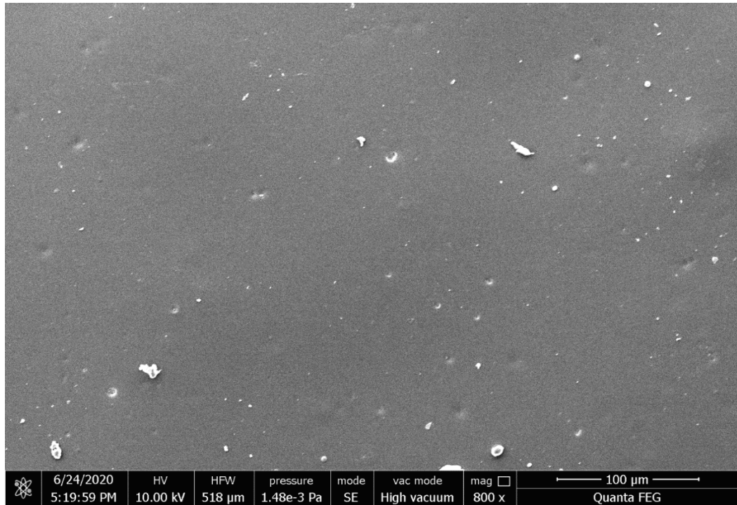
Şekil 5.2 Modifiyesiz (kontrol) D70 vernik katmanı SEM görüntüsü
