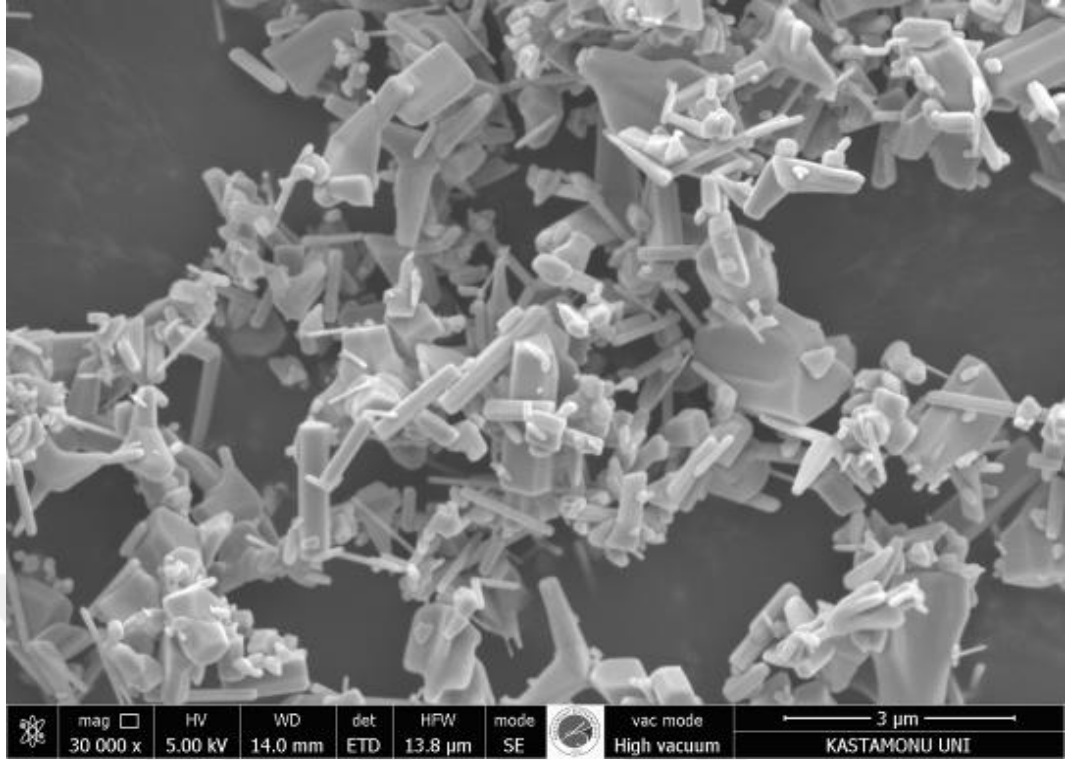
Şekil 3.2 Çinko oksitin 30 000 kat büyütülmüş SEM görüntüsü
