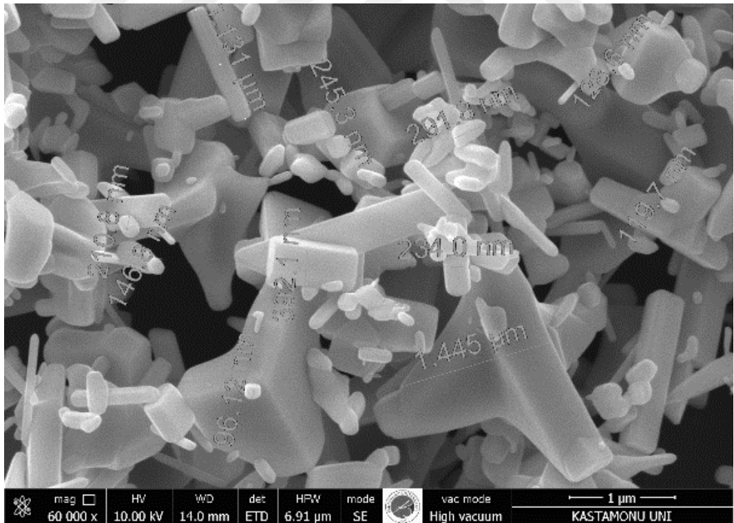
Şekil 3.3 Çinko oksitin 60 000 kat büyütülmüş SEM görüntüsü
