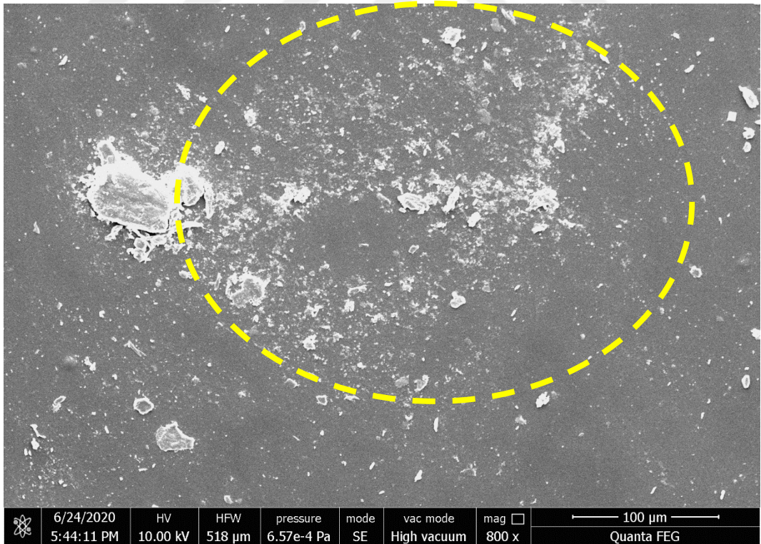
Şekil 5.8 D99 vernik katmanında ZnO'in 2 nolu SEM görüntüsü
