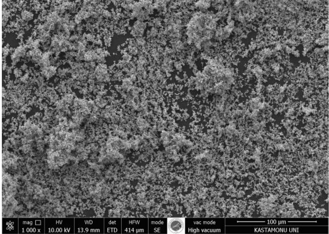
Şekil 3.1 Çinko oksitin 1000 kat büyütülmüş SEM görüntüsü
