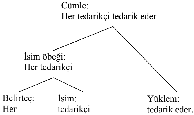
Şekil 3.7. Bir cümlenin söz dizim analizi
