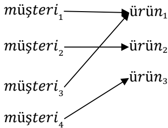
Şekil 3.10. Müşteri ve ürün kümeleri arasındaki satın alma bağıntısı
