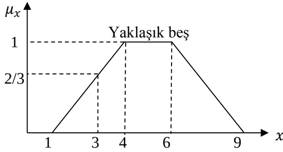
Şekil 3.5. ‘Yaklaşık beş’ yamuk üyelik fonksiyonu
