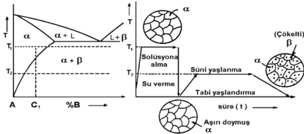
Şekil 6.3. Yaşlandırma ısıtma işlemi için faz diyagramına göre sıcaklıkların gösterimi
