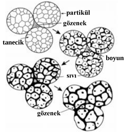
Resim 5.7. Süperkatı üzeri sıvı faz sinterleme işleminin şematik görünümü
