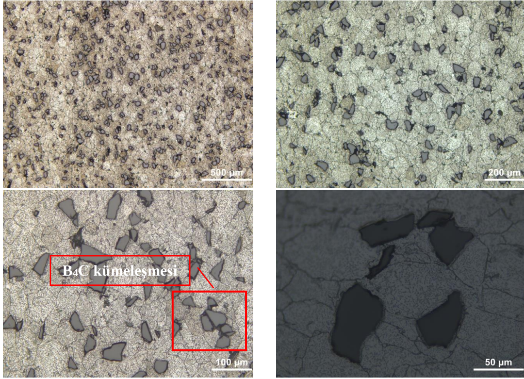
Resim 9.9. 610S-10 MMK p numunesinin farklı büyütme oranlarındaki mikroyapı görüntüleri
