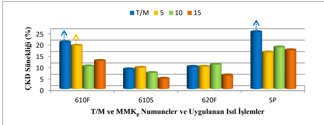
Şekil 9.5. T/M ve MMK p malzemelerin süneklik değerlerinin karşılaştırılması
