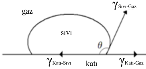
Resim 3.1. Islatma durumları için katı-sıvı-gaz denge koşulları şematik gösterimi
