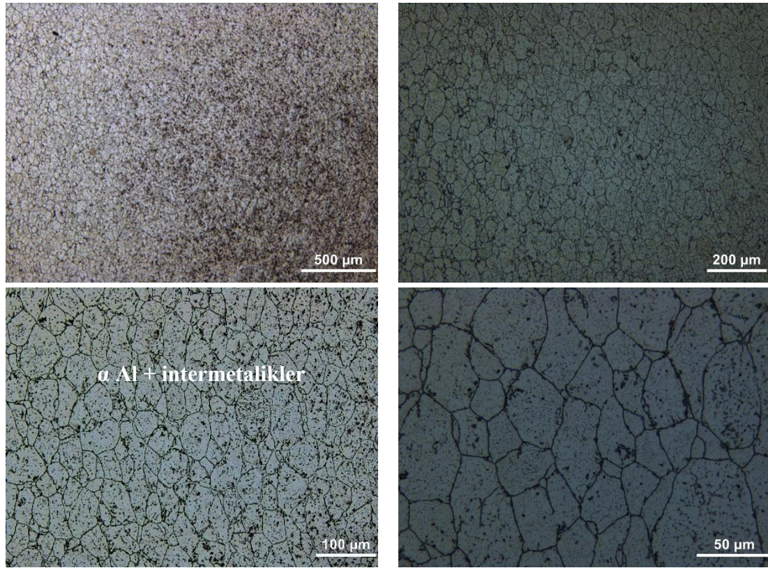
Resim 9.3. SP-T/M numunesinin farklı büyütme oranlarındaki mikroyapı görüntüleri
