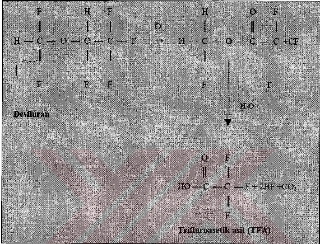
Şekil 3. Desfluranın metabolizması
