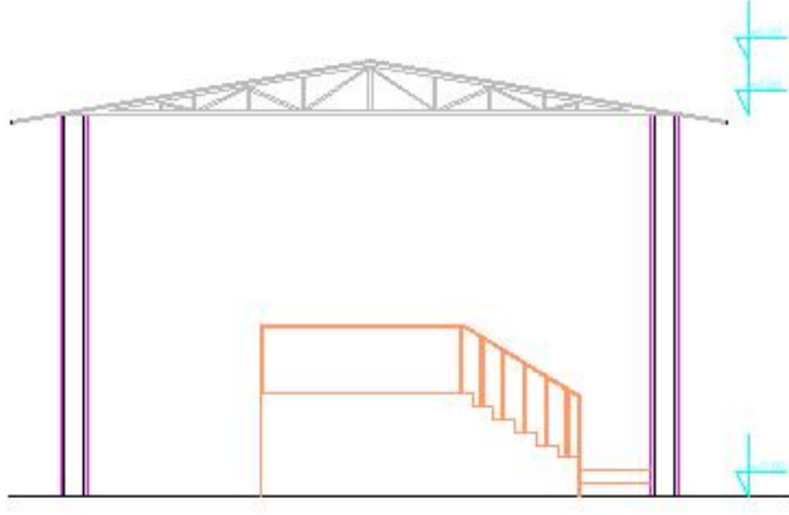
Şekil 2.10 Araç Yıkama Ünitesi Kesiti
