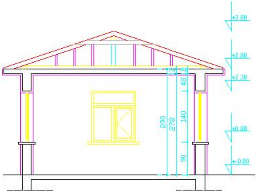
Şekil 2.3 Kantar Binası Kesiti
