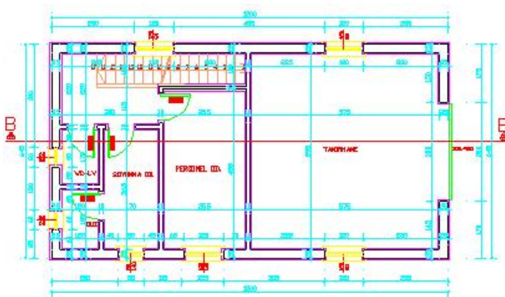
Şekil 2.17 Tamirhane Üst Kat Planı
