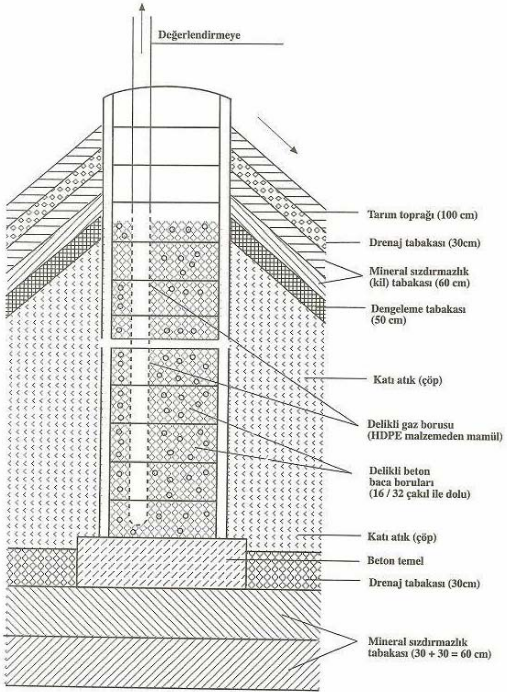
Şekil 9.5. Gaz Toplama Bacası [8]
