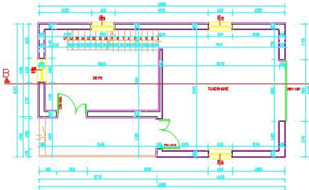
Şekil 2.16 Tamirhane Alt Kat Planı
