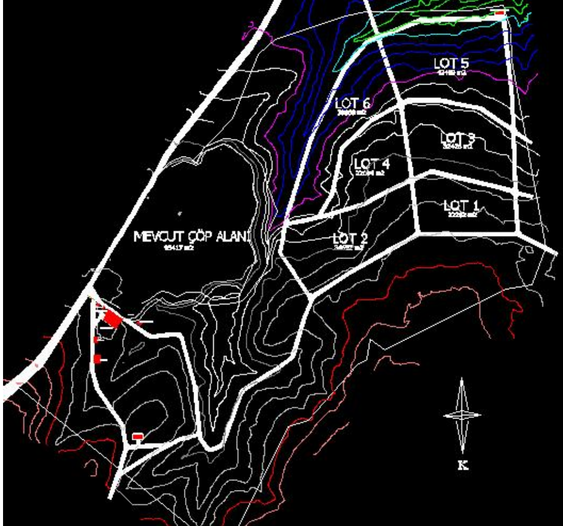
Şekil 1.3 Katı Atık Düzenli Depolama Alanı Vaziyet Planı
