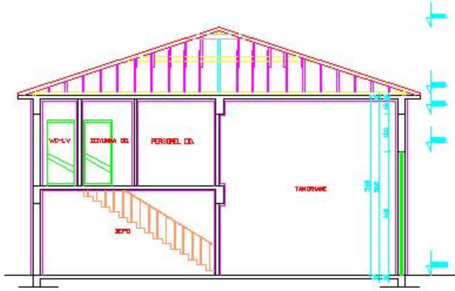
Şekil 2.18 Tamirhane Kesiti
