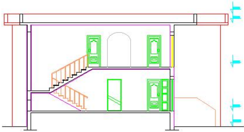
Şekil 2.14 İdari Bina Kesiti
