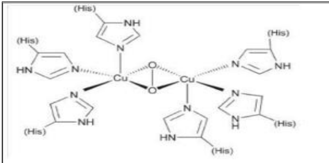
Şekil 2.7. Tirozinaz enziminin aktif bölgesi (Garcia-Molina, 2007).
